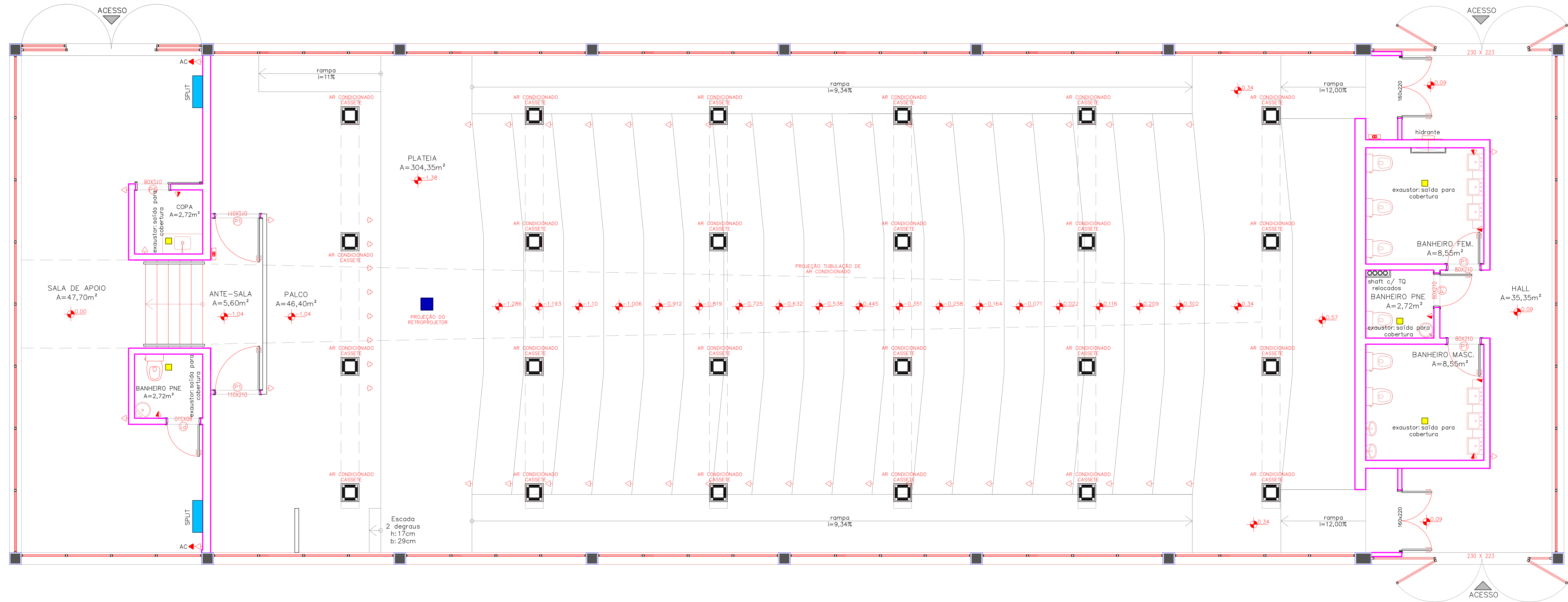
PLANTA DE INFRAESTRUTURA Escala 1/50
