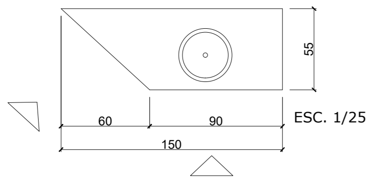
BALCÃO 3 - VISTA FRONTAL FECHADO
