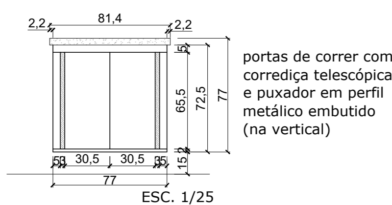
BALCÃO 3 - VISTA LATERAL FECHADO
