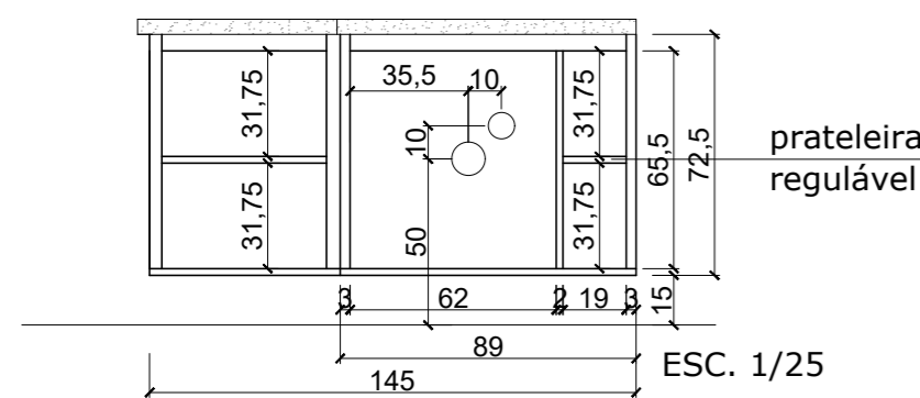
BALCÃO 3 - VISTA FRONTAL ABERTO
