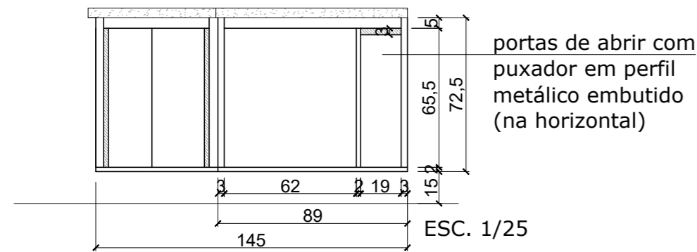
BALCÃO 3 - VISTA FRONTAL ABERTO
