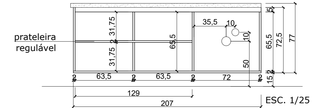
BALCÃO 5 - VISTA FRONTAL ABERTO
