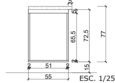
BALCÃO 4 - VISTA LATERAL
