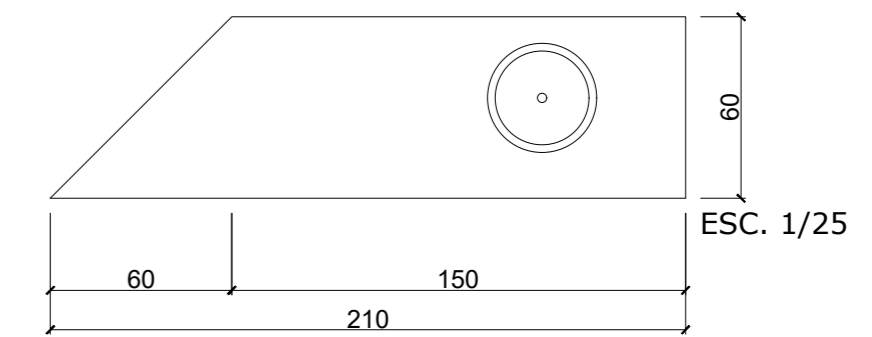
BALCÃO 5 - PLANTA BAIXA
