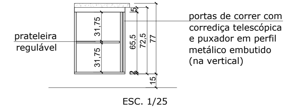
BALCÃO 5 - VISTA LATERAL
