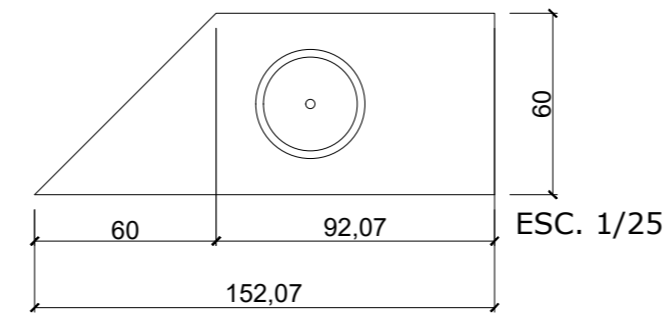
BALCÃO 4 - PLANTA BAIXA
