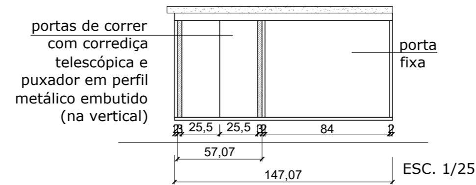
BALCÃO 4 - VISTA FRONTAL FECHADO
