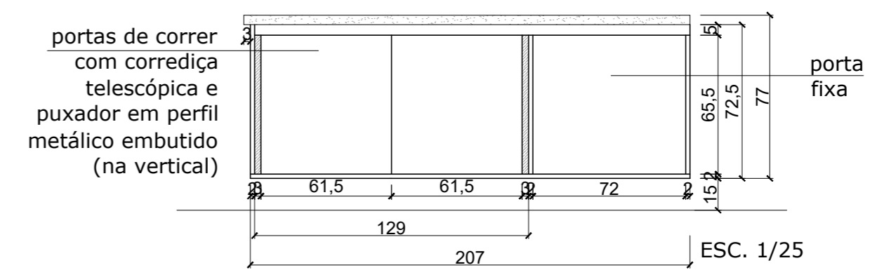
BALCÃO 5 - VISTA FRONTAL FECHADO
