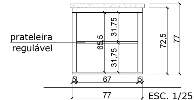
BALCÃO 3 - VISTA LATERAL ABERTO
