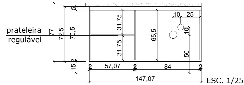
BALCÃO 4 - VISTA FRONTAL ABERTO
