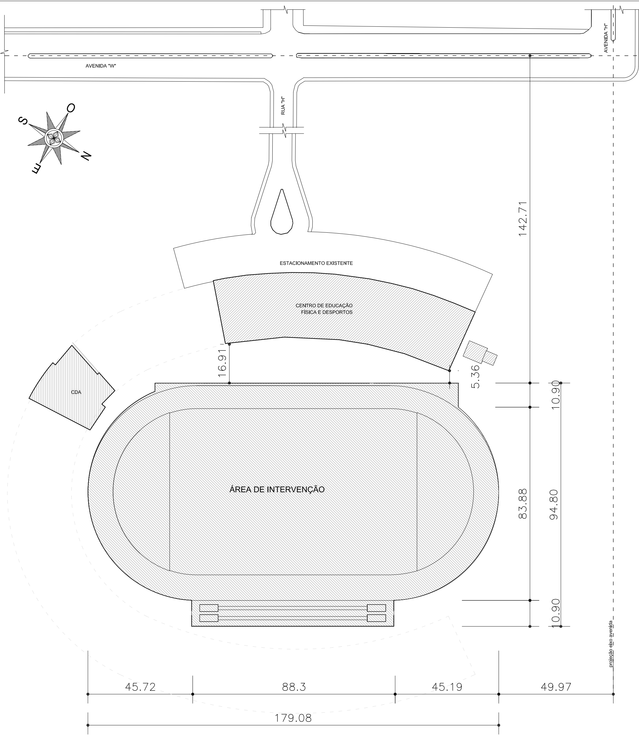
Situação Escala: 1/1000
