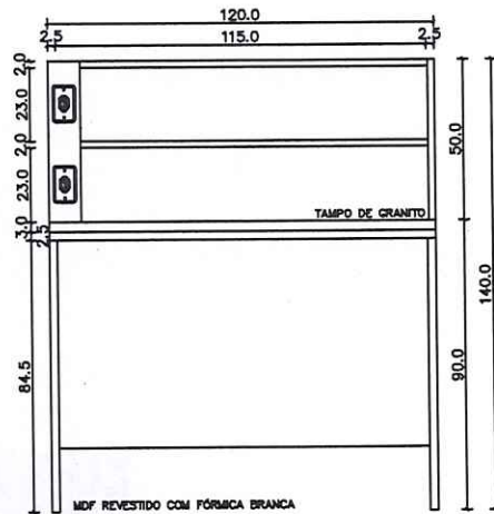
Corte Longitudinal Escala 1:25
