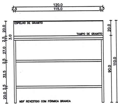
Corte Longitudinal Escala 1:25
