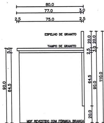
Corte Transversal Escala 1:25
