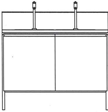
Vista Frontal Escala 1:25
