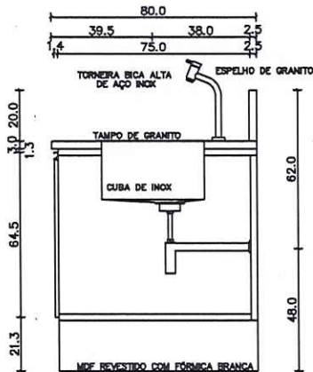
Corte Transversal Escala 1:25
