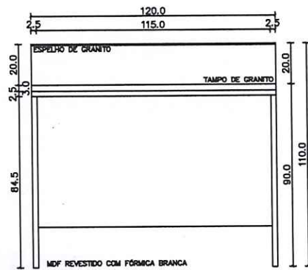
Corte Longitudinal Escala 1:25
