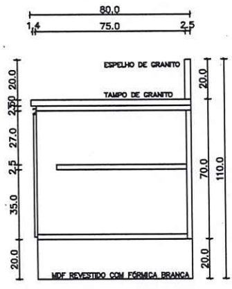
Corte Transversal Escala 1:25
