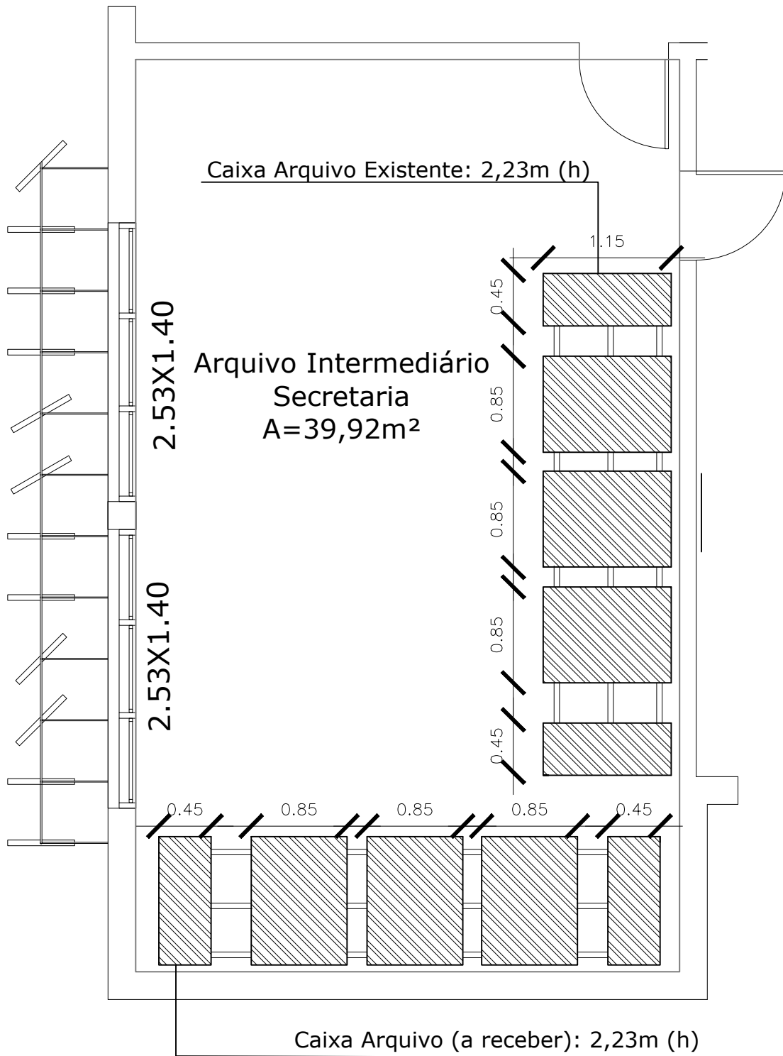
Distribuição de Mobiliário- Layout
