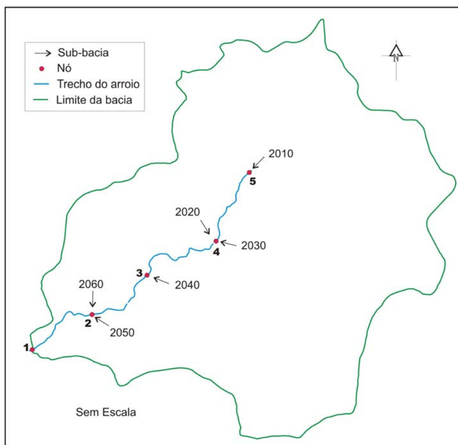
FIGURA 23 – Concepção dos canais e sub-bacias para a simulação simplificada
