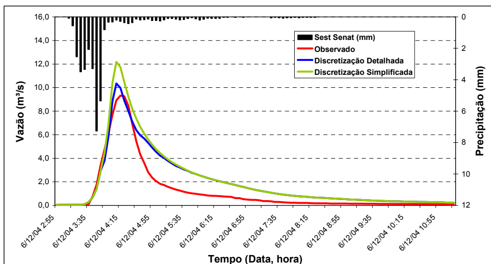
FIGURA 37 – Evento do dia 06/12/2004 - condição de escoamento B
