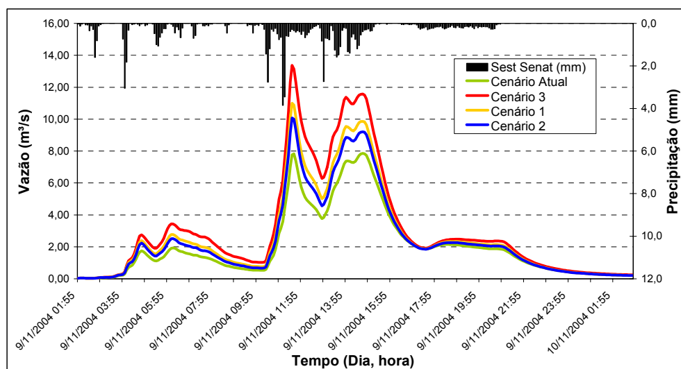
FIGURA 57 – Hidrogramas do evento do dia 11/09/2004, para os cenários de urbanização
