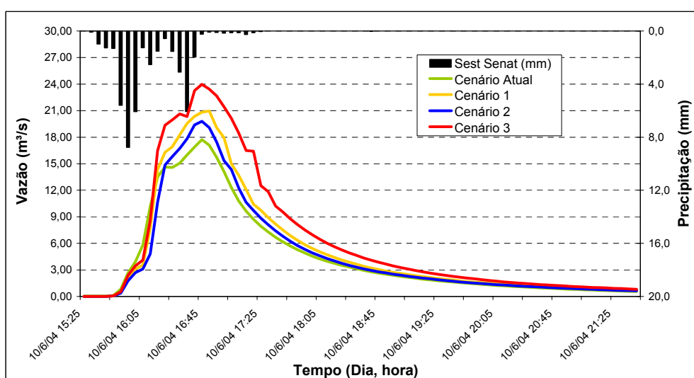
FIGURA 56 – Hidrogramas do evento do dia 10/06/2004, para os cenários de urbanização
