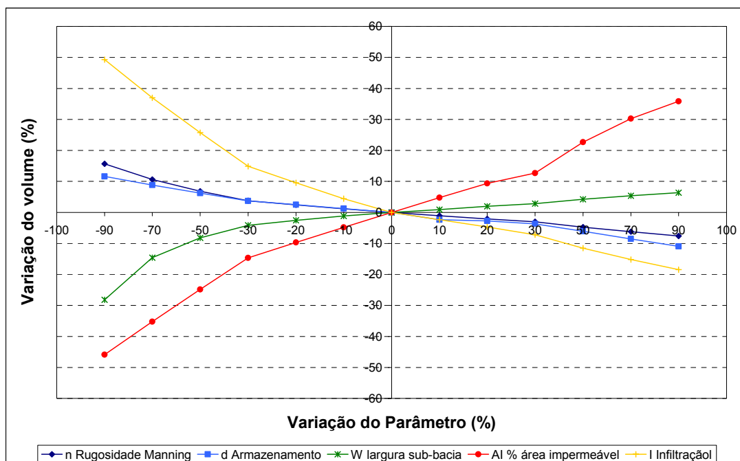
FIGURA 46 – Influência dos parâmetros do módulo Runoff no volume escoado
