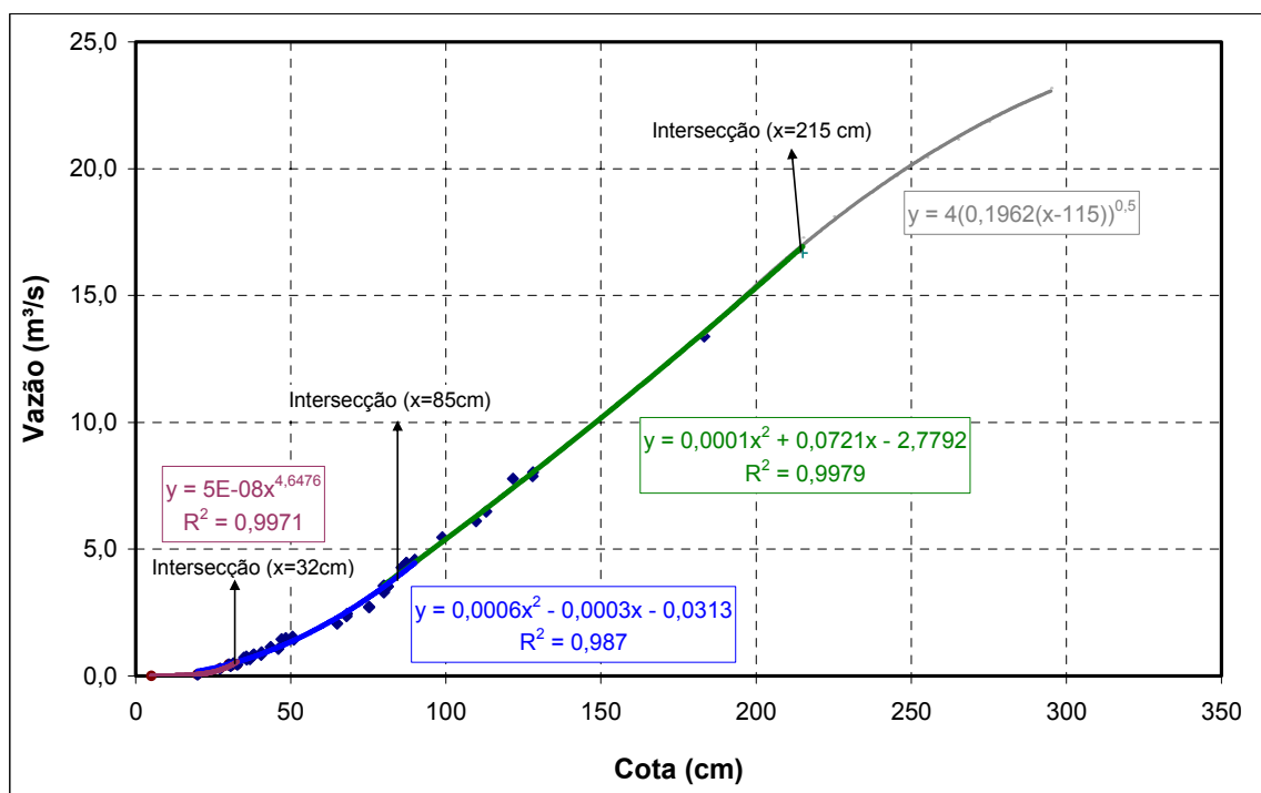
FIGURA 17 – Curva chave determinada no período de monitoramento
