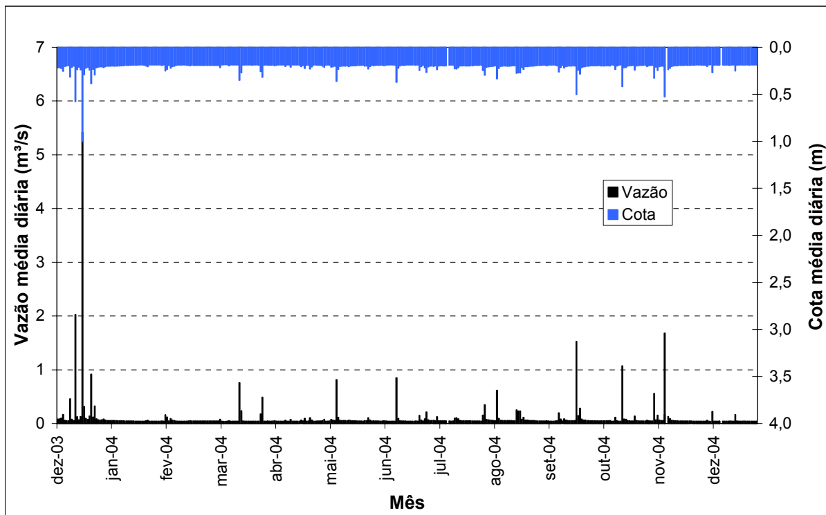
FIGURA 15 – Vazões e cotas médias observadas na estação fluviográfica Canela
