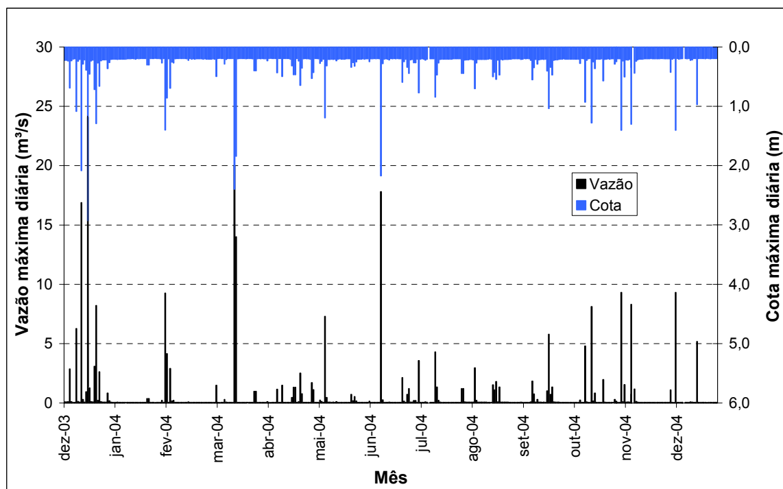
FIGURA 16 – Vazões e cotas máximas observadas na estação fluviográfica Canela
