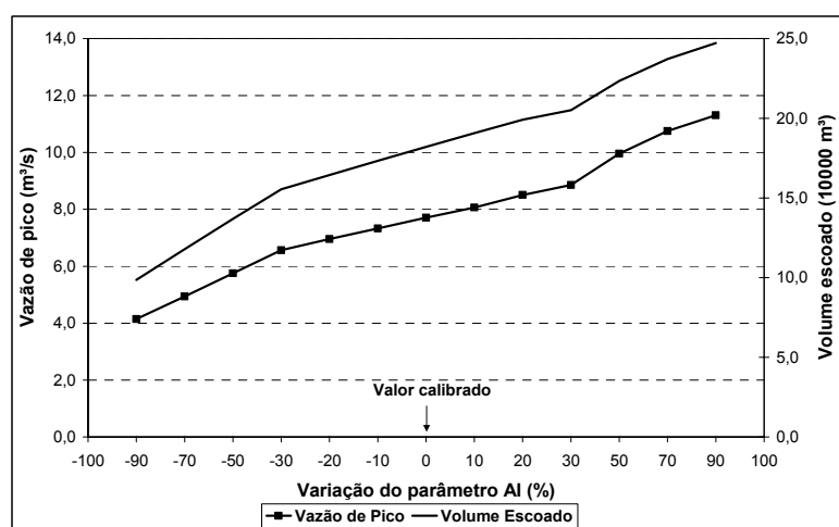
FIGURA 47 – Influência do parâmetro AI na vazão de pico e no volume escoado
