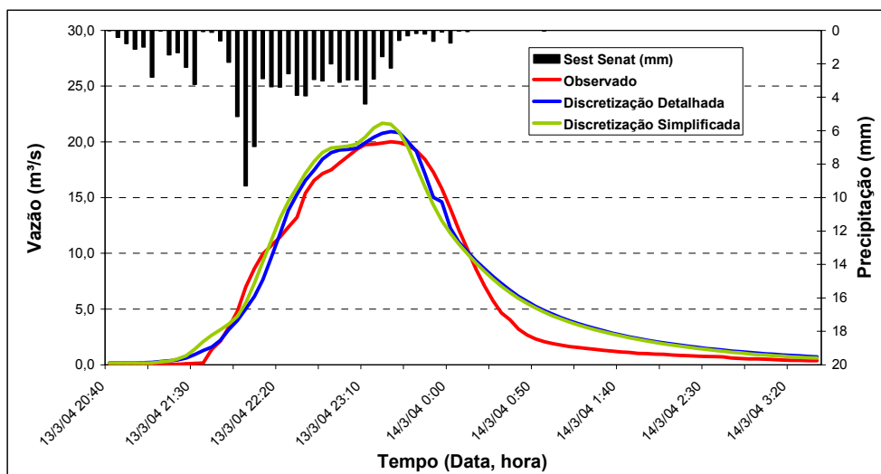
FIGURA 30 – Evento do dia 13/03/2004 - condição de escoamento A
