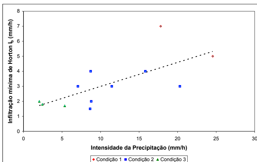
FIGURA 42 – Variação da intensidade média de precipitação em função do I_b
