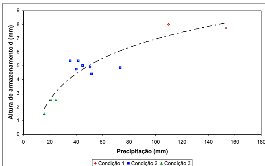
FIGURA 41 – Variação do armazenamento em função da precipitação total do evento
