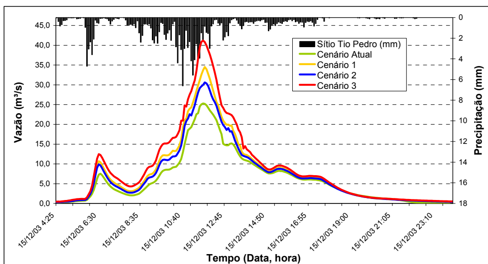
FIGURA 54 – Hidrogramas do evento do dia 15/12/2003, para os cenários de urbanização
