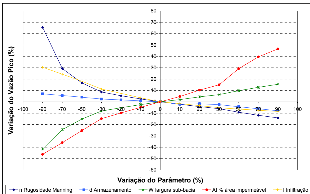
FIGURA 45 – Influência dos parâmetros do módulo Runoff na vazão de pico
