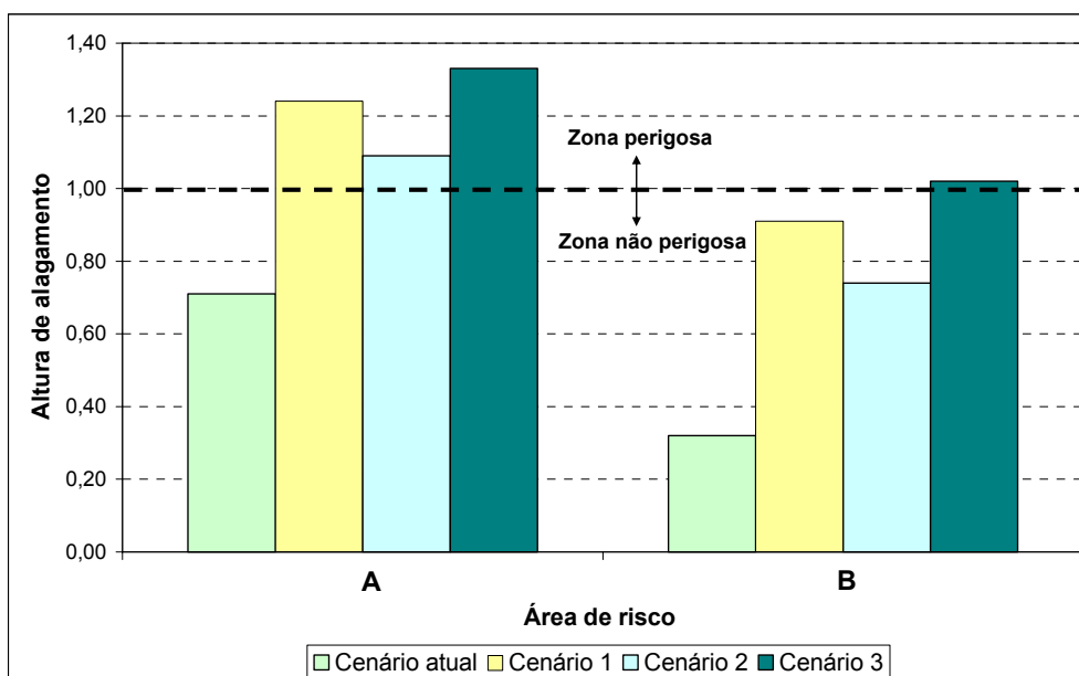
FIGURA 59 – Avaliação das áreas com potencial de risco à população – Evento: 15/12/2003
