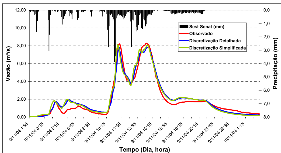
FIGURA 35 – Evento do dia 09/11/2004 - condição de escoamento B
