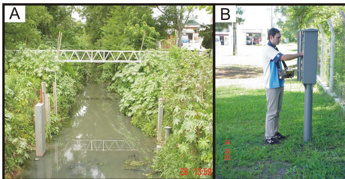
FIGURA 14 – Foto da seção de medição de vazão (A) e obtenção dos dados do registrador de nível (B)
