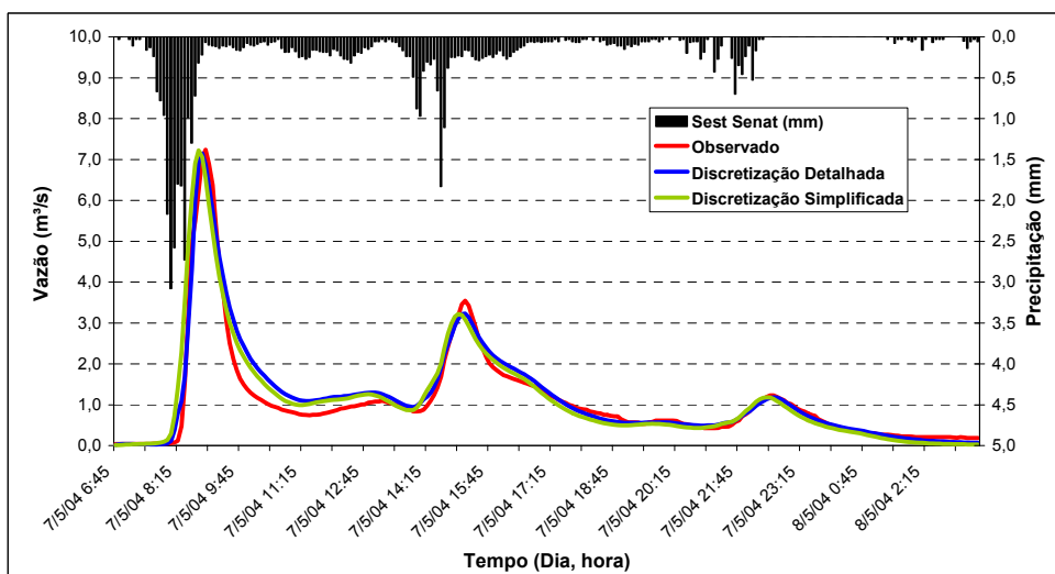
FIGURA 32 - Evento do dia 07/05/2004 - condição de escoamento B
