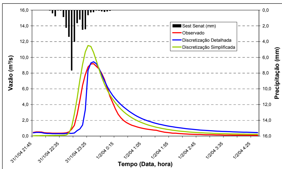
FIGURA 31 – Evento do dia 31/01/2004 - condição de escoamento B
