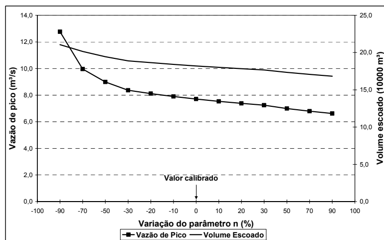
FIGURA 49 – Influência do parâmetro n na vazão de pico e no volume escoado
