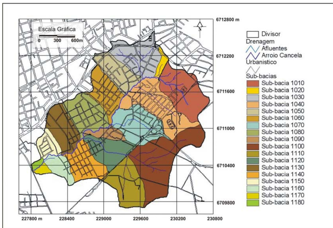
FIGURA 20 – Bacia hidrográfica do Arroio Cancela com discretização detalhada em dezoito sub-bacias
