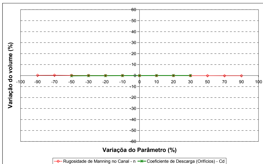
FIGURA 53 – Influência dos parâmetros do módulo Extran no volume escoado
