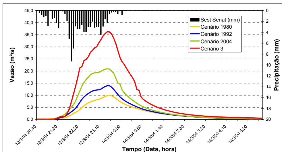
FIGURA 62 – Simulação do evento do dia 13/03/2004, para os anos de 1980, 1992, 2004 e um cenário futuro de urbanização
