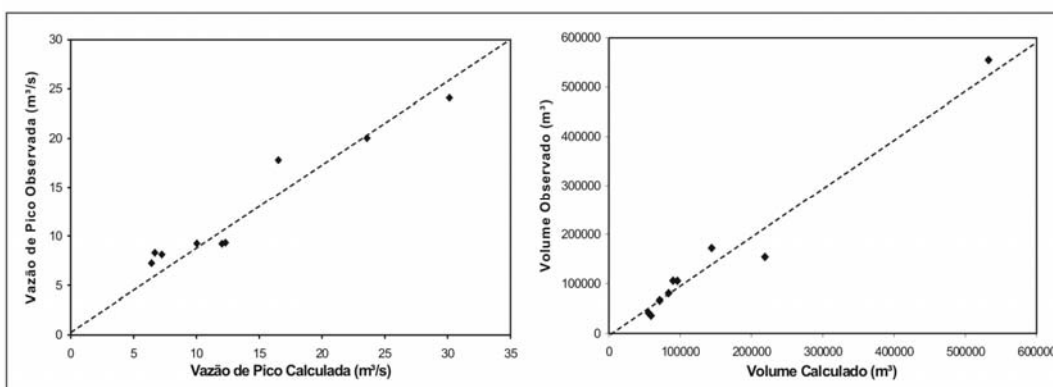
FIGURA 44 – Resultados da vazão de pico e do volume escoado para o conjunto AB, em função dos valores observados
