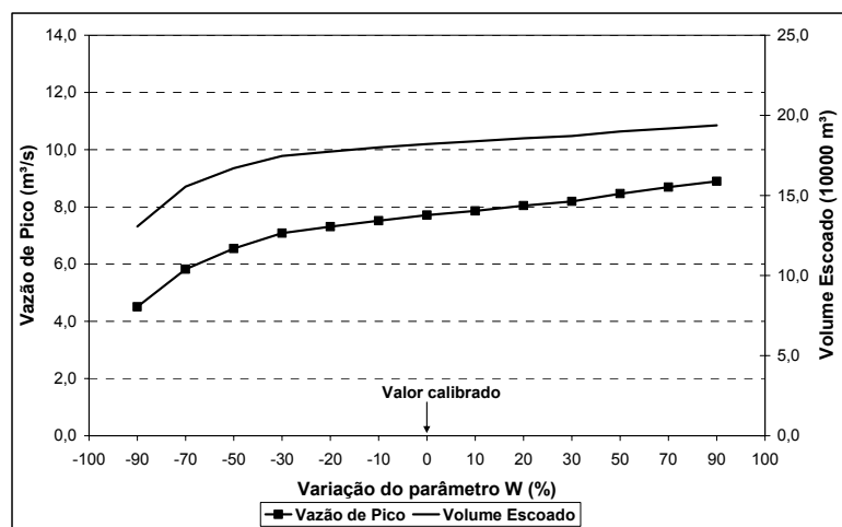
FIGURA 48 – Influência do parâmetro W na vazão de pico e no volume escoado
