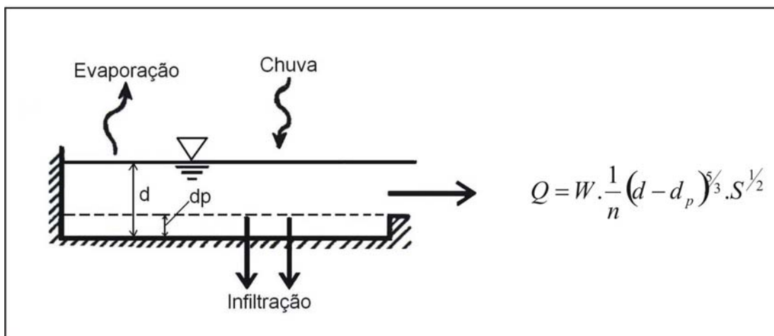
FIGURA 70 – Representação do reservatório não linear das sub-bacias
