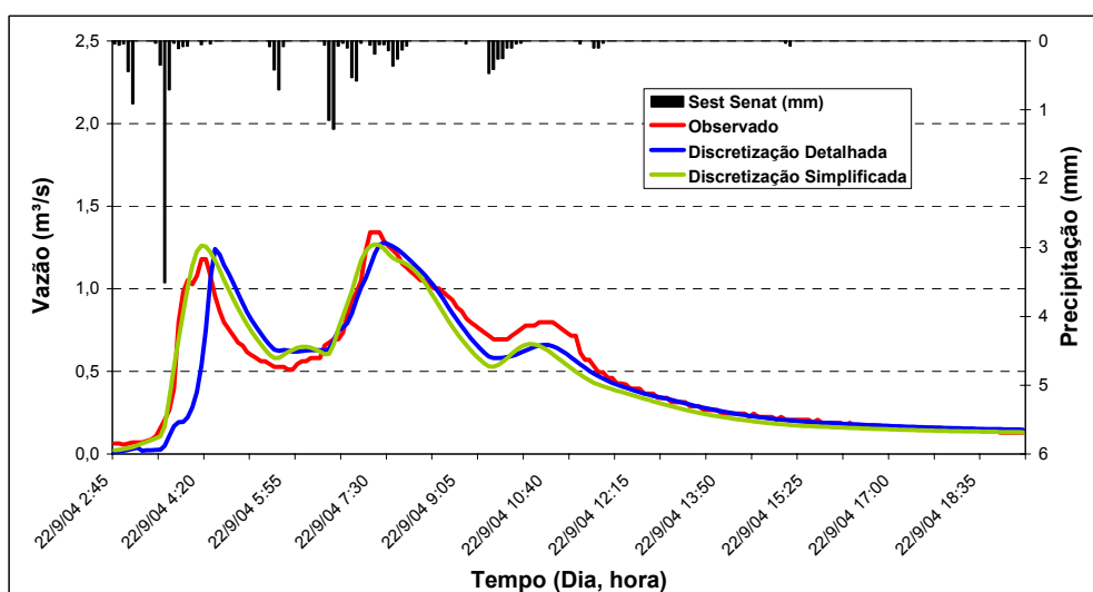
FIGURA 38 – Evento do dia 22/09/2004 - condição de escoamento C
