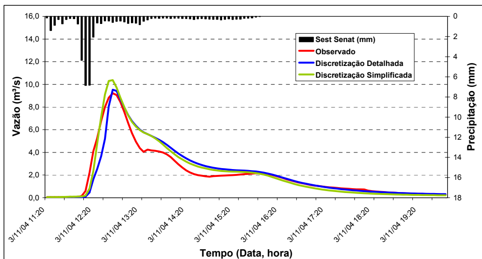
FIGURA 36 – Evento do dia 03/11/2004 - condição de escoamento B
