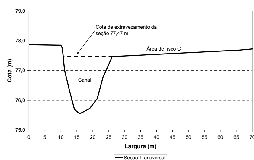
FIGURA 26 – Seção transversal característica do trecho 113
