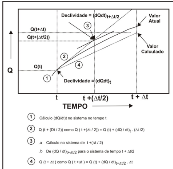
FIGURA 72 – Método de Euler modificado para a descarga baseado nas projeções de t+\Delta t/2 e t+\Delta t . (modificado de James et al., 2003)
