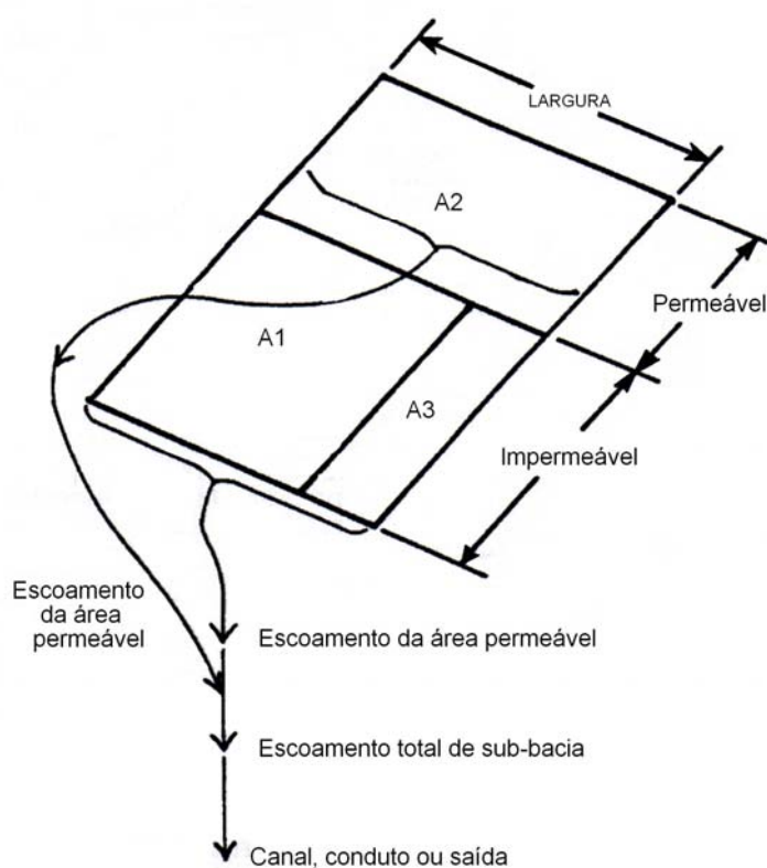
FIGURA 69 – Esquemática das sub-bacias
