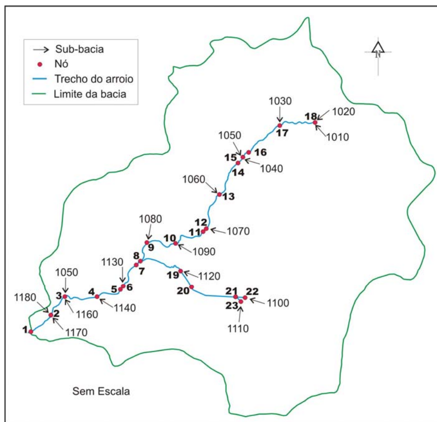
FIGURA 22 – Concepção dos canais e sub-bacias para a simulação detalhada
