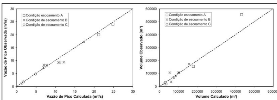
FIGURA 43 – Resultados da vazão de pico e do volume escoado para os conjuntos A, B e C, em função dos valores observados
