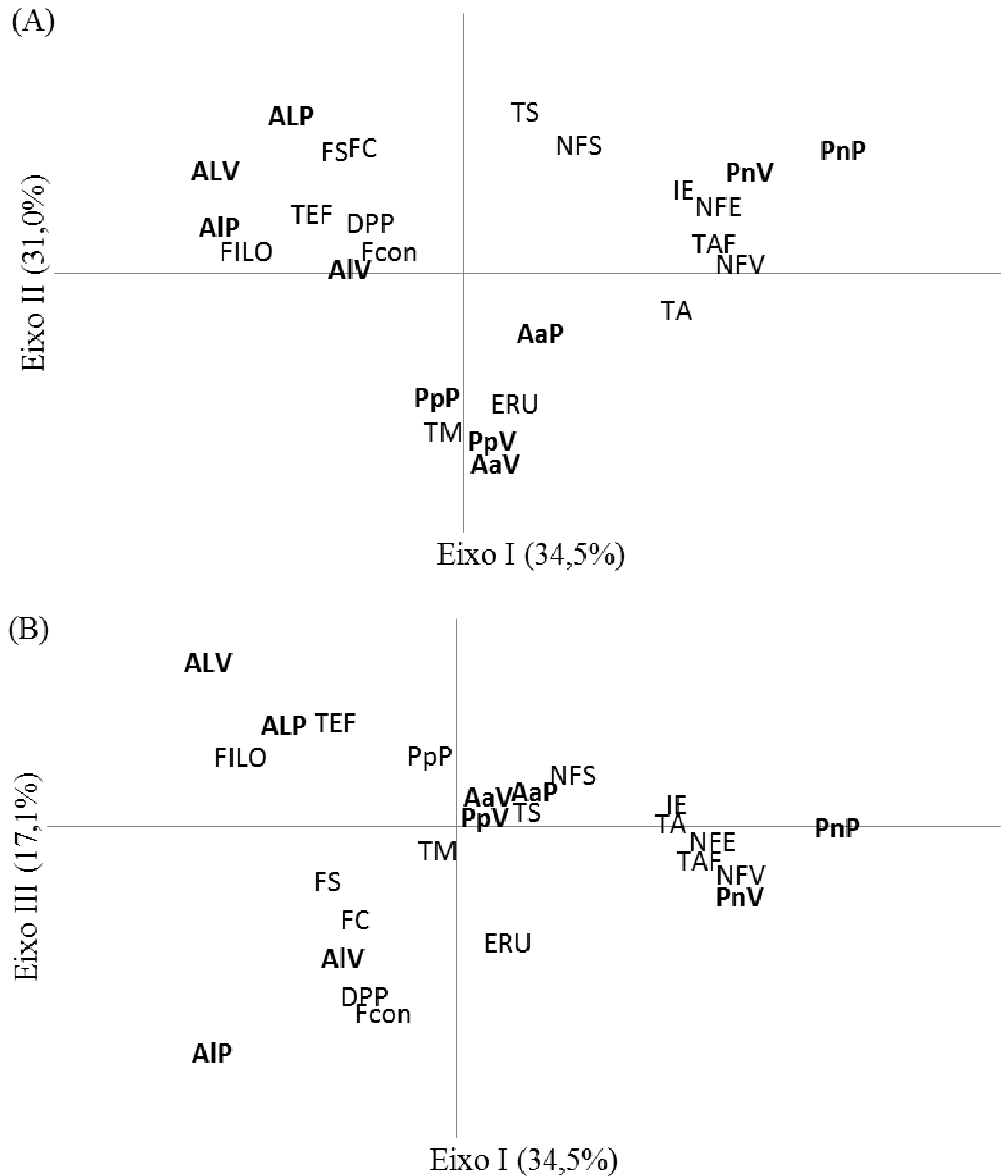
Figura 2 - Diagrama de ordenação, por coordenadas principais, das variáveis morfológicas, fluxos de tecido foliar e demografia de perfilhamento das espécies avaliadas segundo as estações do ano. As espécies e as variáveis estão dispostas no plano de ordenação, de acordo com suas correlações com os eixos I, II e III. Legenda das espécies: Aa = Axonopus affinis , Al = Andropogon lateralis , AL = Aristida laevis , Pn = Paspalum notatum e Pp = Paspalum plicatulum . Legenda das estações: P = primavera de 2010; V = verão de 2011. Legenda das variáveis: DPP= densidade populacional de perfilhos; ERU= eficiência real de utilização; FC= fluxo de crescimento foliar; Fcon= fluxo de consumo foliar; FILO= filocrono; FS= fluxo de senescência foliar; IE= índice de estabilidade da população de perfilhos; NFE= número de folhas em expansão; NFS= número de folhas em senescência; NFV= número de folhas verdes; TA= taxa de aparecimento de perfilhos; TAF = taxa de
