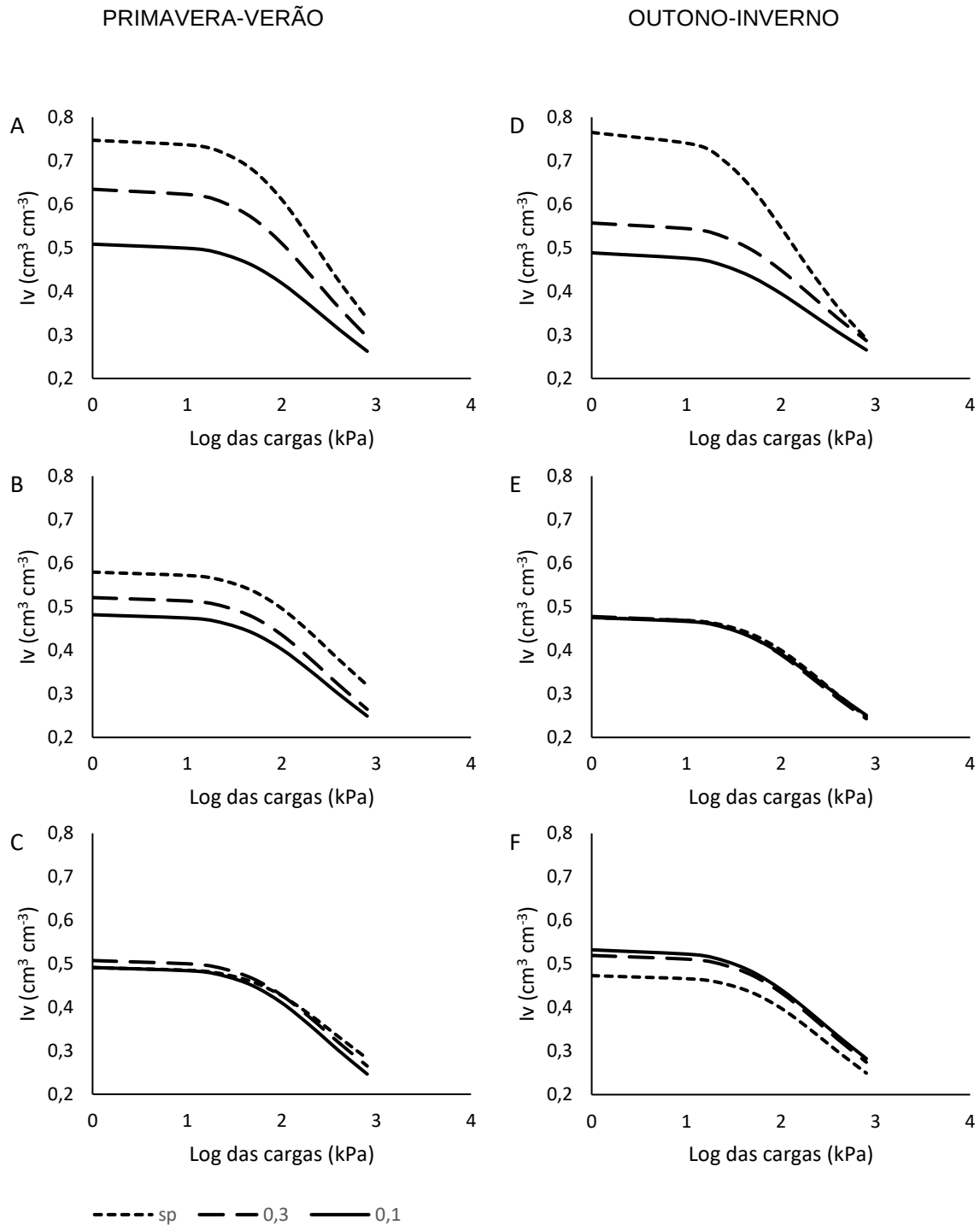
Figura 7 - Curvas de compressão do solo para os períodos primavera-verão e outono-inverno.
