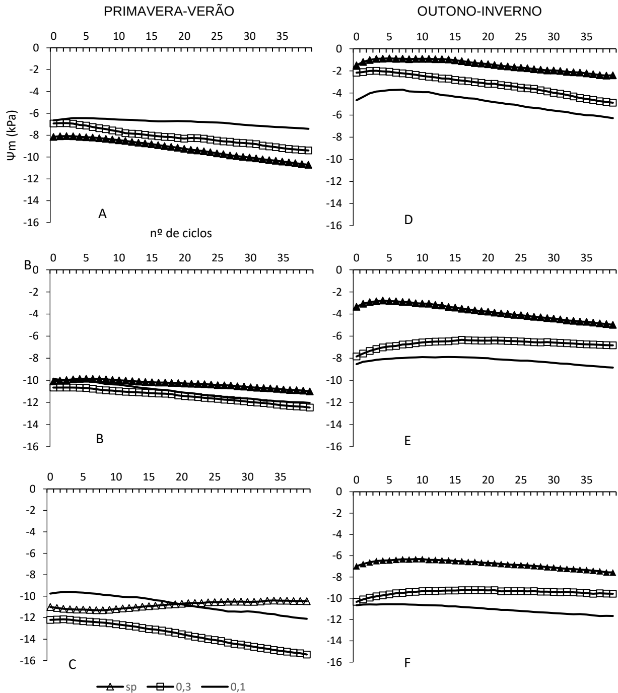
Figura 9 - Variação do potencial matricial ( \Psi_m ) em função dos ciclos de carregamento/descarregamento, para os períodos primavera-verão e outono-inverno as camadas
