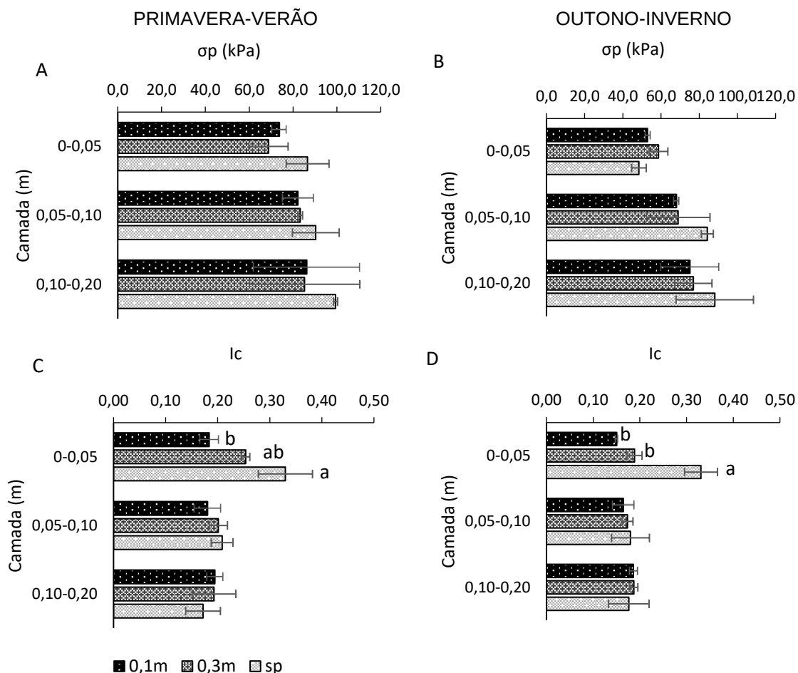
Figura 5 - Valores médios de pressão de preconsolidação (kPa) e índice de compressão para os períodos primavera-verão e outono-inverno.
