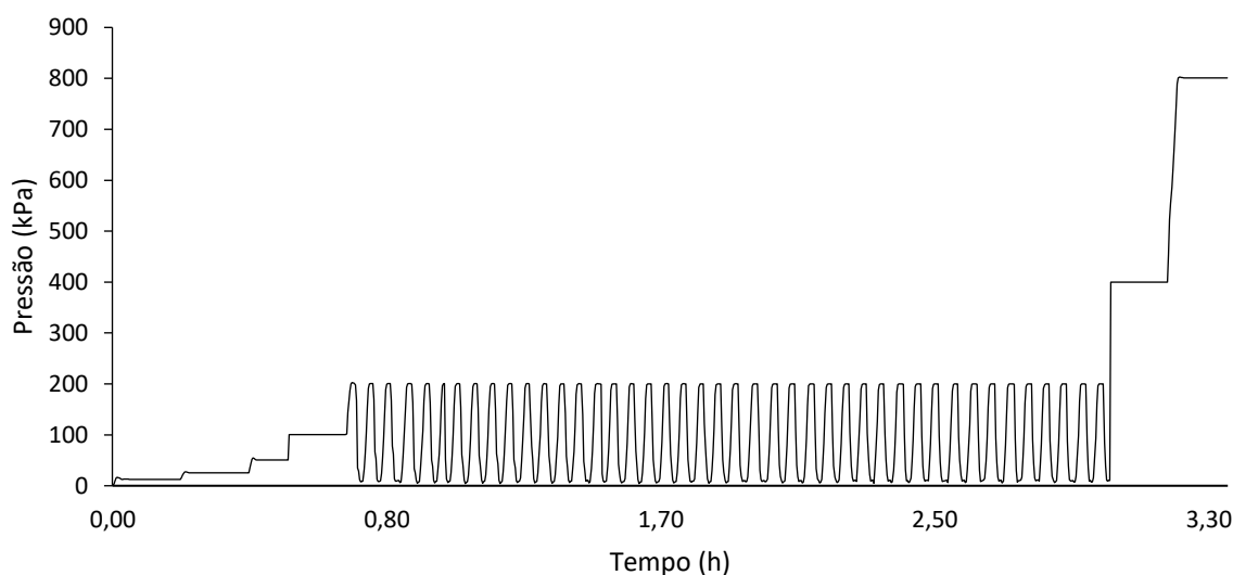
Figura 2 - Relação entre a pressão aplicada na amostra com o tempo de teste no de ensaio de compressão das amostras de solo.
