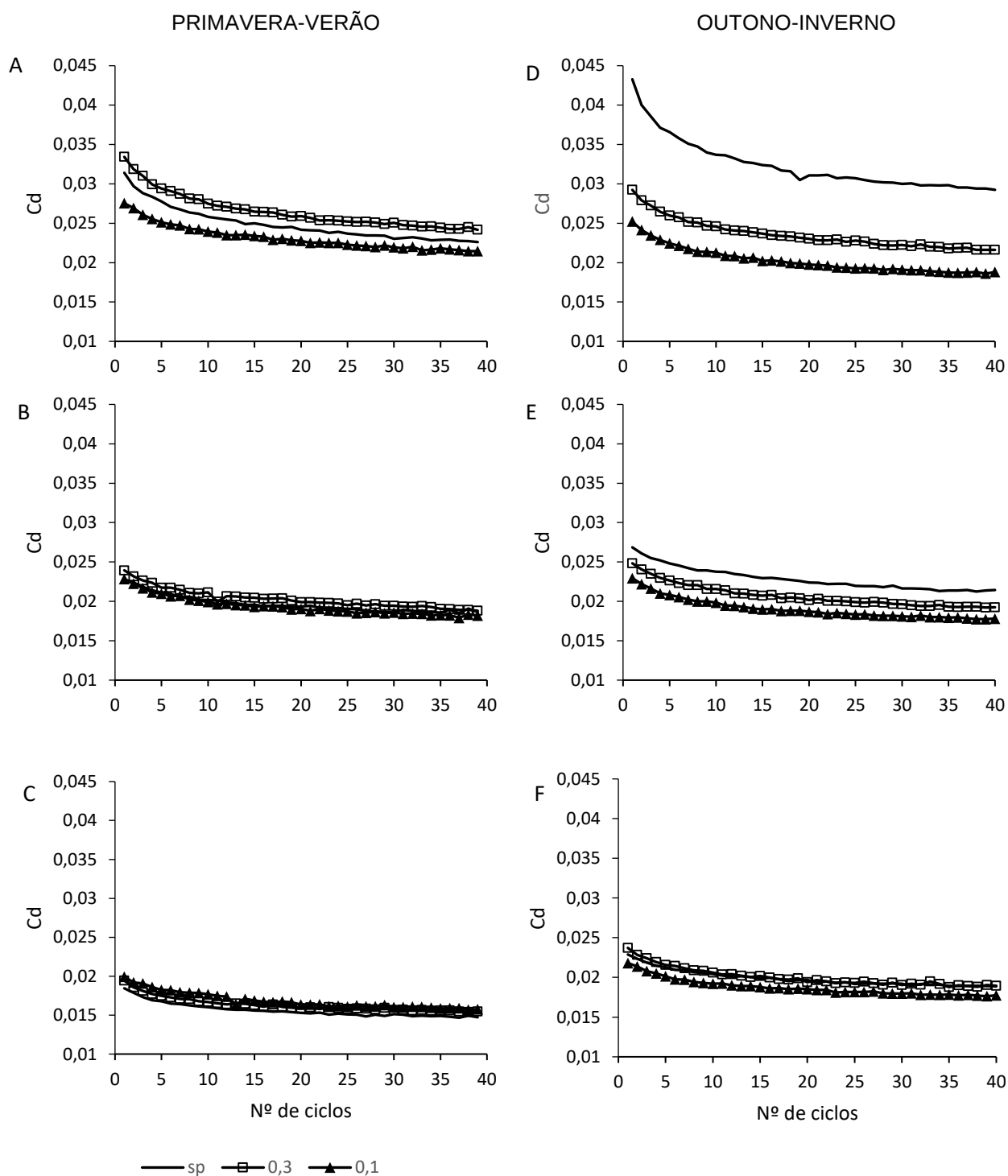
Figura 8 - Variação do coeficiente de descompressão ( C_d ) em função dos ciclos de carregamento/descarregamento, para os períodos primavera-verão e outono-inverno.
