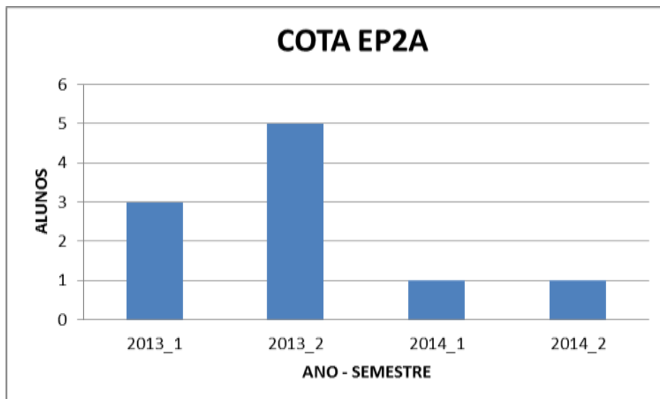
Figura 36 - NÚMERO DE ALUNOS COTISTAS EP2A –MATEMATICA 2008/1 -2014/2
