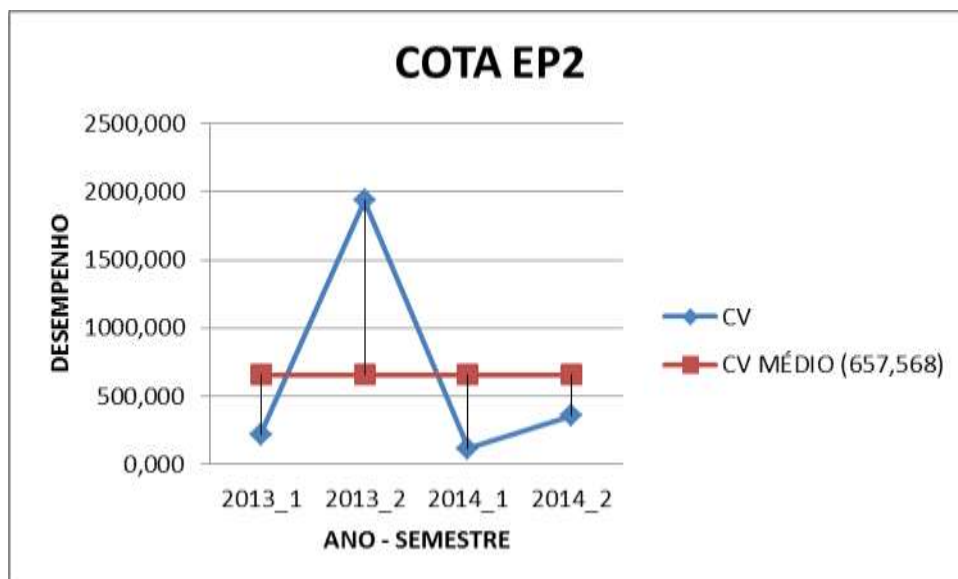
Figura 34 - COEFICIENTE DE VARIAÇÃO DO DESEMPENHO MÉDIO DOS COTISTAS EP2 - ENGENHARIA CIVIL 2009/1 – 2014/2
