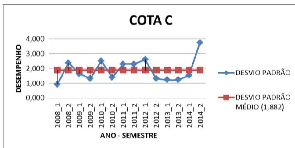
Figura 10 - DESVIO PADRÃO DO DESEMPENHO MÉDIO DOS COTISTAS C - ENGENHARIA CIVIL 2009/1 – 2014/2
