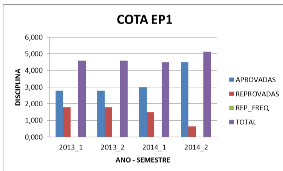
Figura 14- MÉDIA DO NÚMERO MÉDIO DE DISCIPLINAS DOS COTISTAS EP1 - MATEMATICA 2008/1 -2014/2
