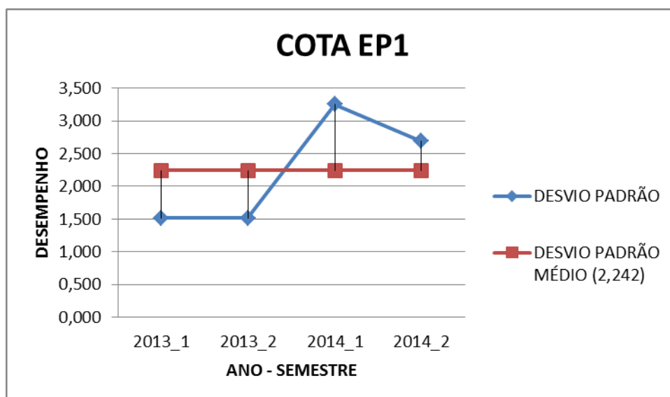
Figura 17 - DESVIO PADRÃO DO DESEMPENHO MÉDIO DOS COTISTAS EP1 –MATEMATICA 2008/1 -2014/2
