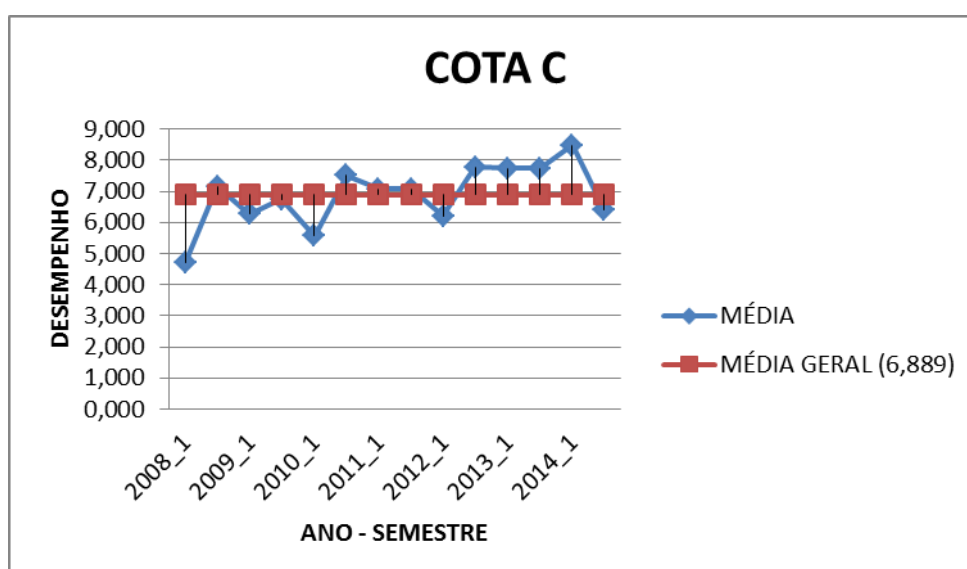
Figura 8 - MÉDIA DO DESEMPENHO MÉDIO DOS COTISTAS C - MATEMATICA 2008/1 -2014/2
