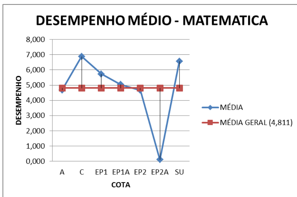
Figura 46 - MÉDIA DO DESEMPENHO MÉDIO PELAS COTAS - MATEMATICA 2008/1 -2014/2
