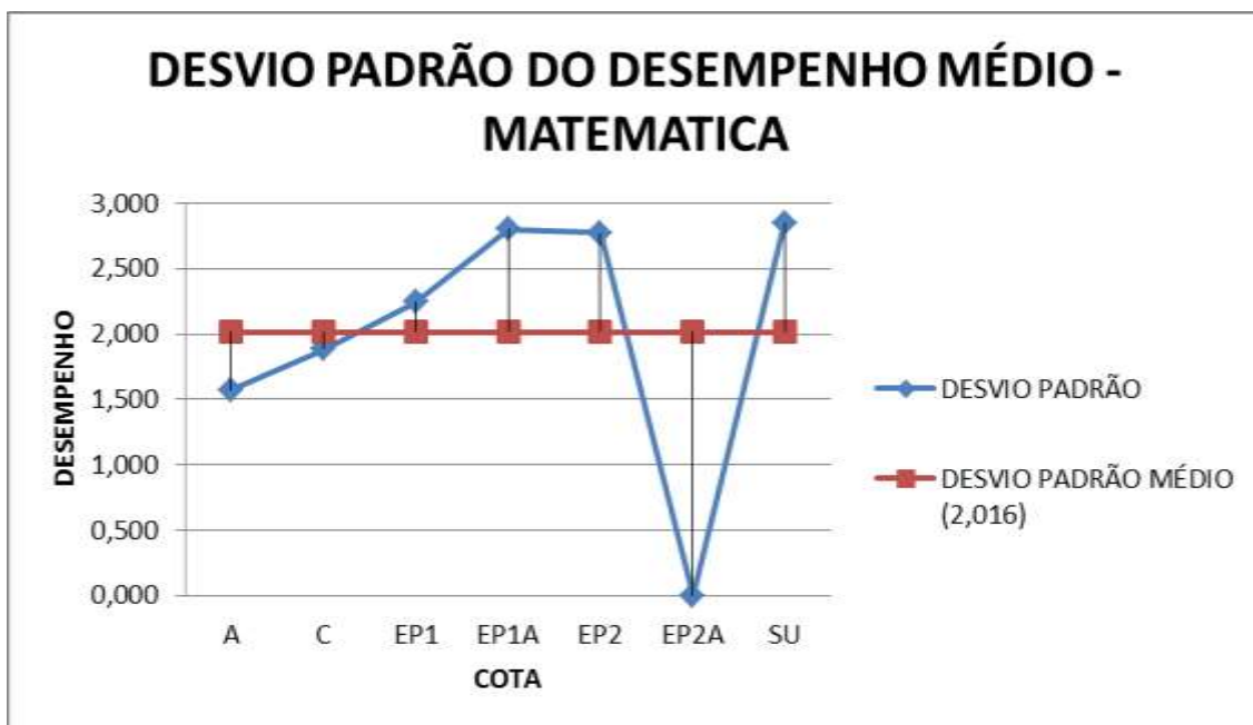
Figura 47 - DESVIO PADRÃO DO DESEMPENHO MÉDIO PELAS COTAS - ENGENHARIA CIVIL 2009/1 – 2014/2
