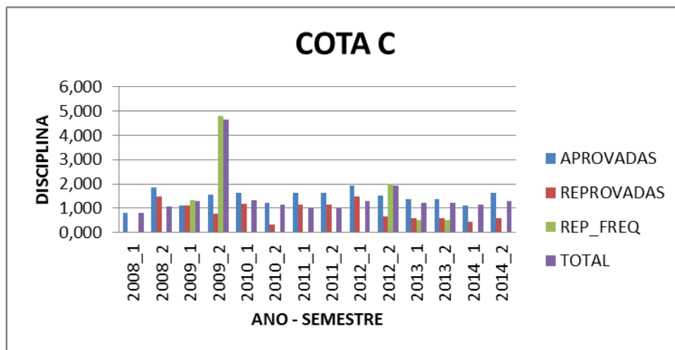
Figura 9 - DESVIO PADRÃO DO NÚMERO MÉDIO DE DISCIPLINAS DOS COTISTAS C – MATEMATICA 2008/1 -2014/2
