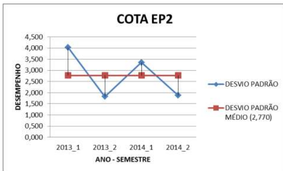
Figura 31 - DESVIO PADRÃO DO DESEMPENHO MÉDIO DOS COTISTAS EP2 –MATEMATICA 2008/1 -2014/2
