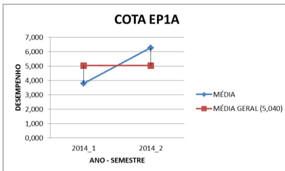
Figura 22 - MÉDIA DO DESEMPENHO MÉDIO DOS COTISTAS EP1A - MATEMATICA 2008/1 - 2014/2
