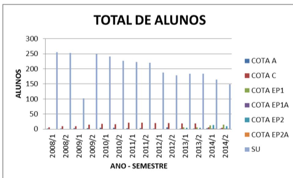
Figura 48 - TOTAL DE ALUNOS PELAS COTAS –MATEMATICA 2008/1 -2014/2
