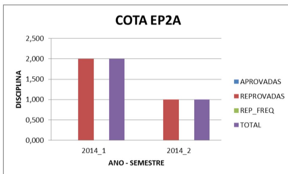
Figura 35- MÉDIA DO NÚMERO MÉDIO DE DISCIPLINAS DOS COTISTAS EP2A –MATEMATICA 2008/1 -2014/2
