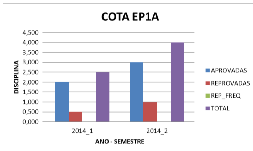
Figura21 - MÉDIA DO NÚMERO MÉDIO DE DISCIPLINAS DOS COTISTAS EP1A - MATEMATICA 2008/1 -2014/2
