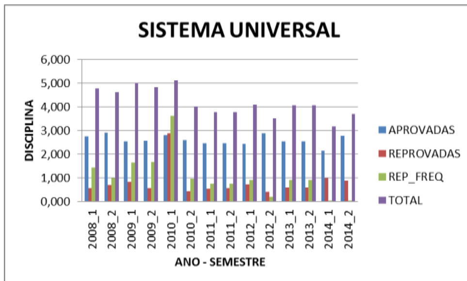
Figura 39 - MÉDIA DO NÚMERO MÉDIO DE DISCIPLINAS DO SISTEMA UNIVERSAL - MATEMATICA 2008/1 -2014/2
