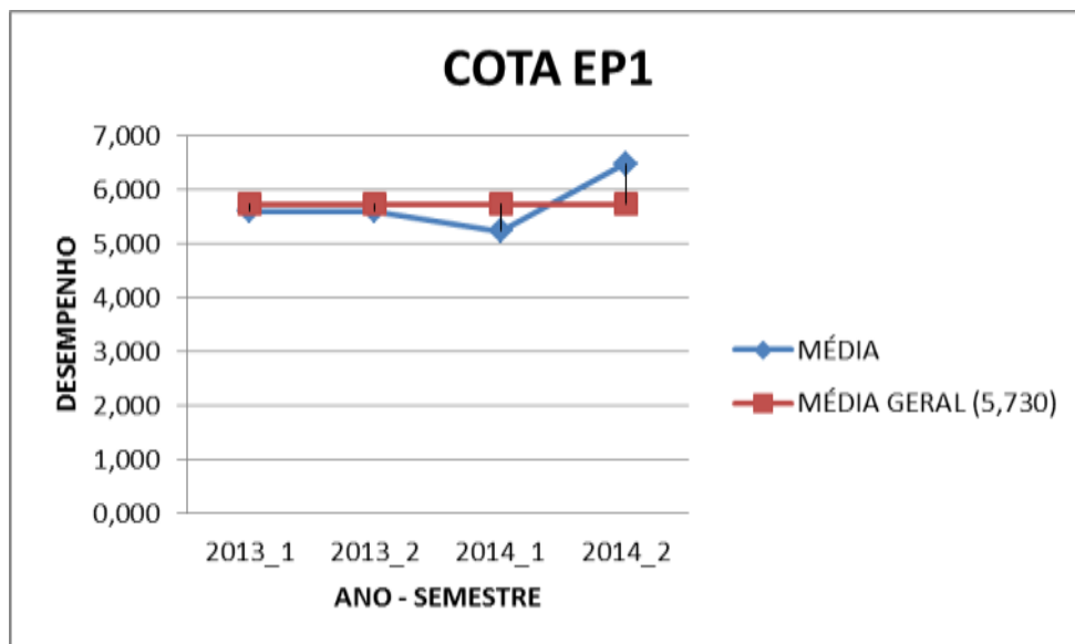
Figura 15 - MÉDIA DO DESEMPENHO MÉDIO DOS COTISTAS EP1 - MATEMATICA 2008/1 - 2014/2
