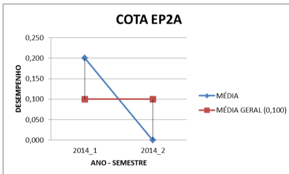
Figura 35 - MÉDIA DO DESEMPENHO MÉDIO DOS COTISTAS EP2A - MATEMATICA 2008/1 - 2014/2
