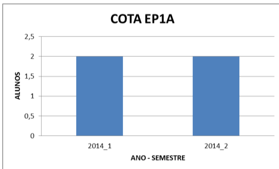
Figura 25 - NÚMERO DE ALUNOS COTISTAS EP1A –MATEMATICA 2008/1 -2014/2
