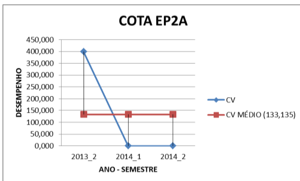
Figura 38 - COEFICIENTE DE VARIAÇÃO DO DESEMPENHO MÉDIO DOS COTISTAS EP2A – MATEMATICA 2008/1 -2014/2
