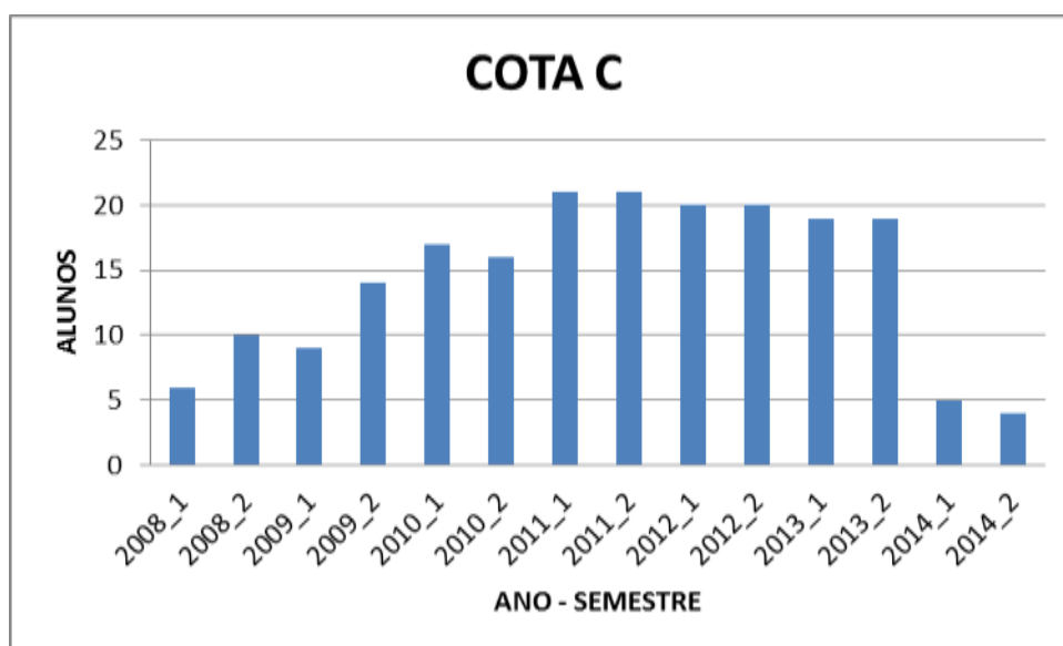
Figura 11- NÚMERO DE ALUNOS COTISTAS C - MATEMATICA 2008/1 -2014/2
