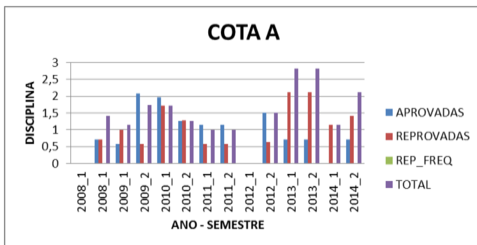
Figura 3 - DESVIO PADRÃO DO NÚMERO MÉDIO DE DISCIPLINAS DOS COTISTAS A - MATEMATICA 2008/1 -2014/2
