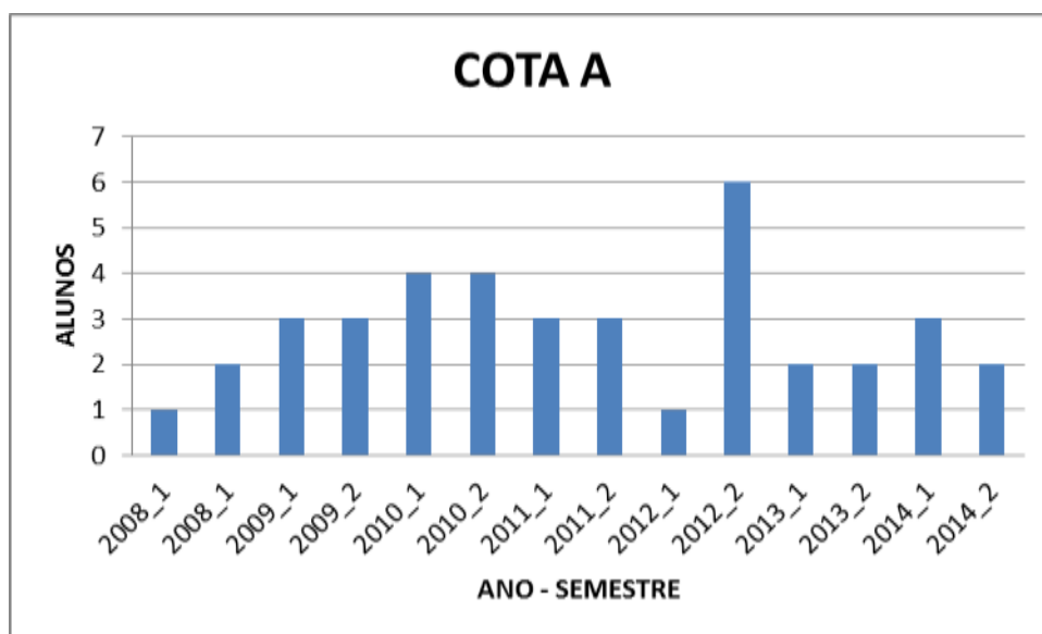
Figura 5 - NÚMERO DE ALUNOS COTISTAS A - MATEMATICA 2008/1 -2014/2
