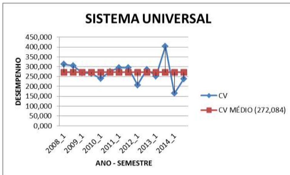
Figura 45 - COEFICIENTE DE VARIAÇÃO DO DESEMPENHO MÉDIO DO SISTEMA UNIVERSAL - ENGENHARIA CIVIL 2009/1 – 2014/2
