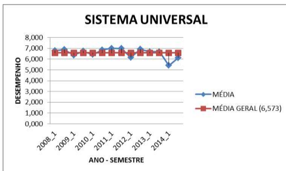
Figura 40 - MÉDIA DO DESEMPENHO MÉDIO DO SISTEMA UNIVERSAL- MATEMATICA 2008/1 -2014/2
