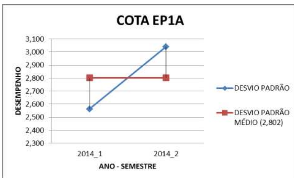
Figura 24- DESVIO PADRÃO DO DESEMPENHO MÉDIO DOS COTISTAS EP1A - MATEMATICA 2008/1 -2014/2
