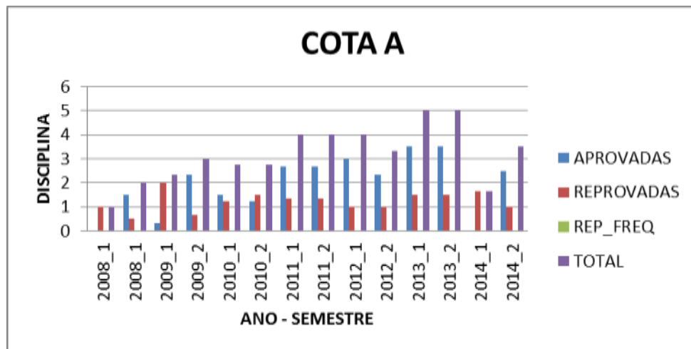
Figura 1 - MÉDIA DO NÚMERO MÉDIO DE DISCIPLINAS DOS COTISTAS A – MATEMATICA 2008/1 -2014/2
