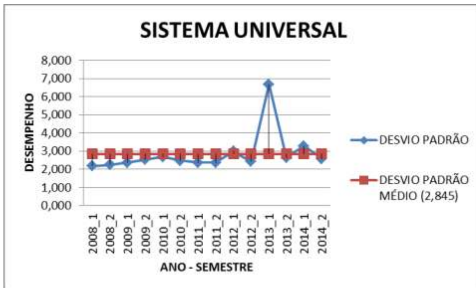
Figura 42 - DESVIO PADRÃO DO DESEMPENHO MÉDIO DO SISTEMA UNIVERSAL - ENGENHARIA CIVIL 2009/1 – 2014/2
