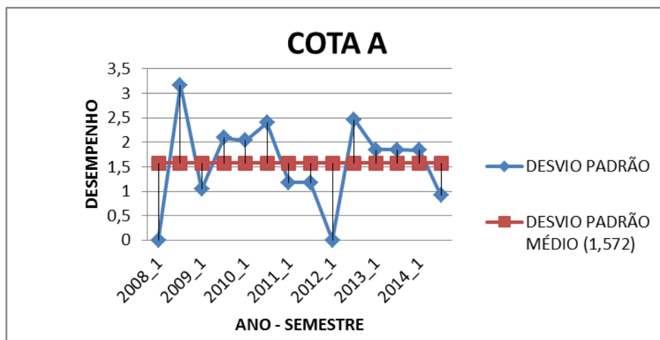
Figura 4 - DESVIO PADRÃO DO DESEMPENHO MÉDIO DOS COTISTAS A MATEMATICA 2008/1 -2014/2
