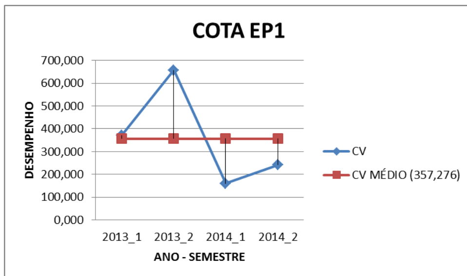
Figura 20 - COEFICIENTE DE VARIAÇÃO DE DESEMPENHO MÉDIO DOS COTISTAS EP1 - ENGENHARIA CIVIL 2009/1 – 2014/2
