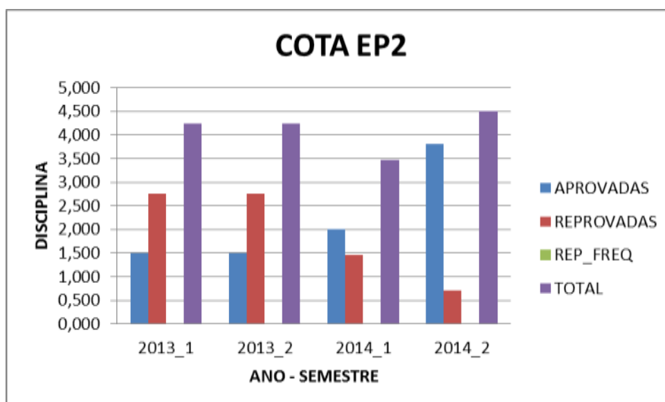
Figura 28 - MÉDIA DO NÚMERO MÉDIO DE DISCIPLINAS DOS COTISTAS EP2 – MATEMATICA 2008/1 -2014/2
