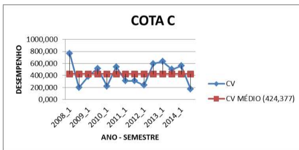
Figura 13 - COEFICIENTE DE VARIAÇÃO DO DESEMPENHO MÉDIO DOS COTISTAS C – ENGENHARIA CIVIL 2009/1 – 2014/2
