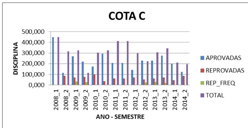
Figura 12- COEFICIENTE DE VARIAÇÃO DO NÚMERO MÉDIO DE DISCIPLINAS DOS COTISTAS C - ENGENHARIA CIVIL 2009/1 – 2014/2
