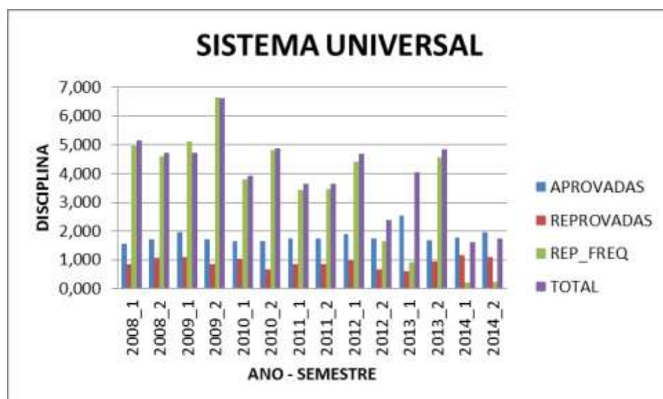
Figura 41 – DESVIO PADRÃO DO NÚMERO MÉDIO DE DISCIPLINAS DO SISTEMA UNIVERSAL - MATEMATICA 2008/1 -2014/2
