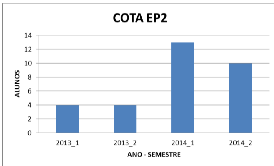
Figura 32 - NÚMERO DE ALUNOS COTISTAS EP2 –MATEMATICA 2008/1 -2014/2
