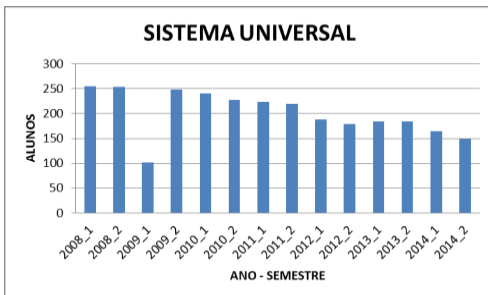
Figura 43 - NÚMERO DE ALUNOS DO SISTEMA UNIVERSAL - MATEMÁTICA 2008/1 -2014/2
