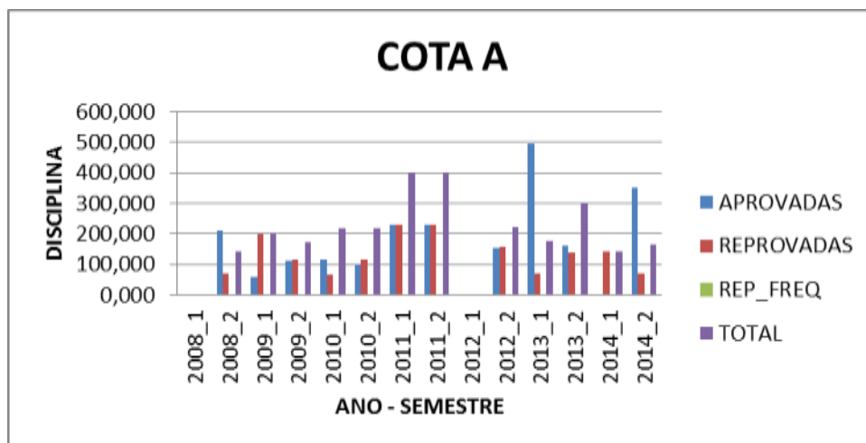
Figura 6 - COEFICIENTE DE VARIAÇÃO DO NÚMERO MÉDIO DE DISCIPLINAS DOS COTISTAS A - MATEMATICA 2008/1 -2014/2
