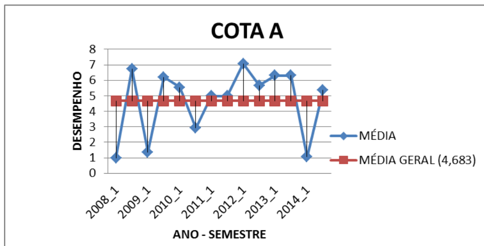
Figura 2 - MÉDIA DO DESEMPENHO MÉDIO DOS COTISTAS A – MATEMATICA 2008/1 -2014/2
