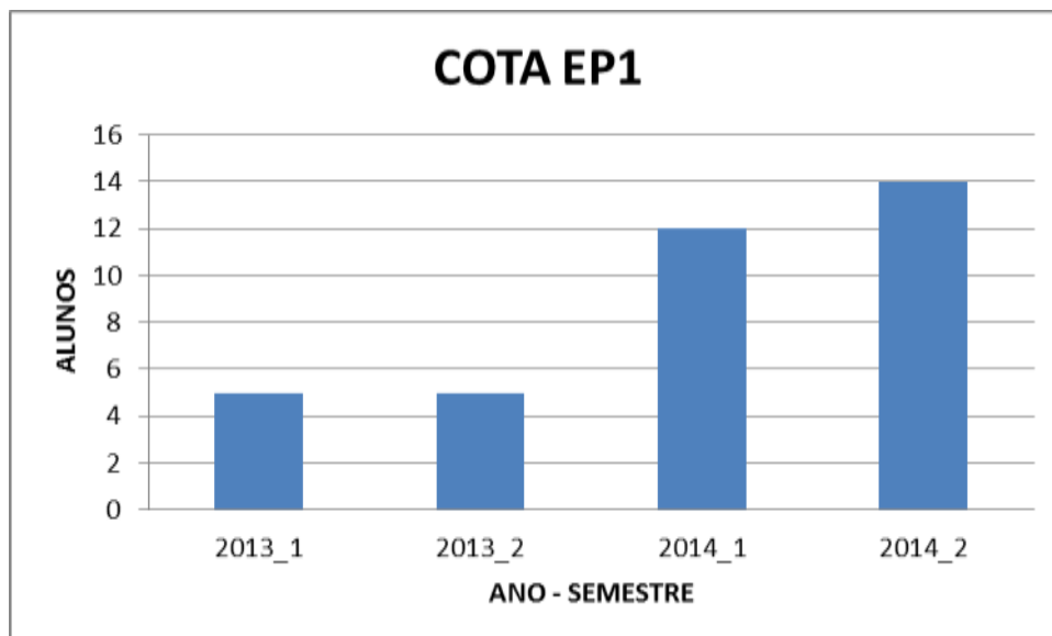
Figura 18 - NÚMERO DE ALUNOS COTISTAS EP1 - MATEMATICA 2008/1 -2014/2
