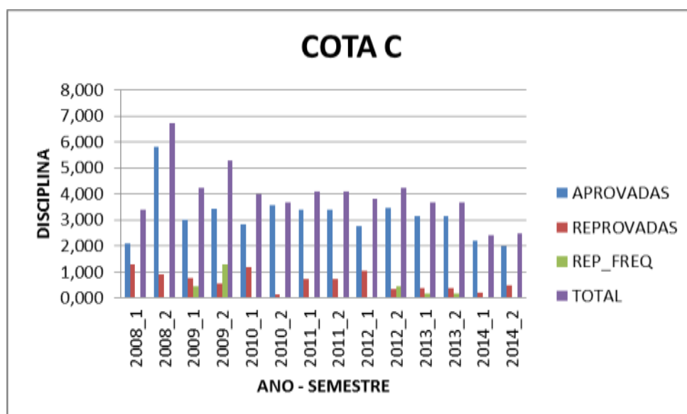
Figura 7 – MÉDIA DO NÚMERO MÉDIO DE DISCIPLINAS DOS COTISTAS C - ENGENHARIA CIVIL 2009/1 – 2014/2
