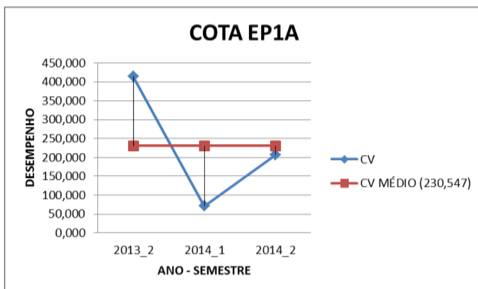
Figura27- COEFICIENTE DE VARIAÇÃO DE DESEMPENHO MÉDIO DOS COTISTAS EP1A –MATEMATICA 2008/1 - 2014/2
