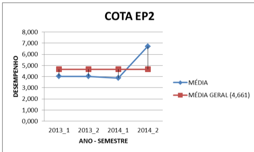
Figura 29 - MÉDIA DO DESEMPENHO MÉDIO DOS COTISTAS EP2 –MATEMATICA 2008/1 - 2014/2
