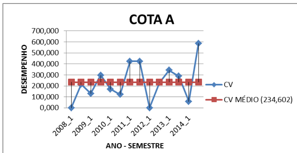
Figura 7 - COEFICIENTE DE VARIAÇÃO DO DESEMPENHO MÉDIO DOS COTISTAS A - MATEMATICA 2008/1 -2014/2
