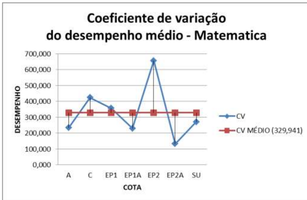
Figura 49 - COEFICIENTE DE VARIAÇÃO DO DESEMPENHO MÉDIO PELAS COTAS - MATEMÁTICA 2008/1 - 2014/2
