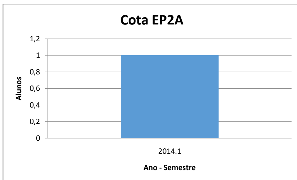
Figura 35 - Número de alunos da Cota EP2A - Química Industrial 2013 a 2014
