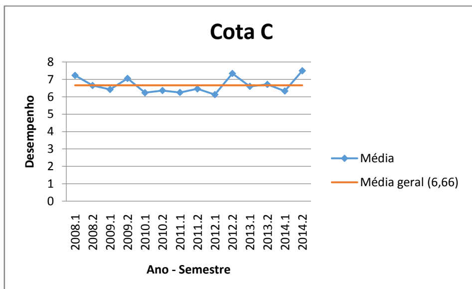
Figura 12 - Média do desempenho médio da Cota C- Química Industrial 2008 a 2014
