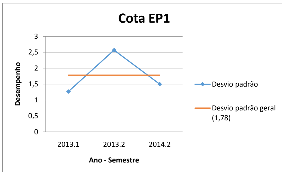
Figura 21 - Desvio padrão do desempenho médio da Cota EP1- Química Industrial 2013 a 2014
