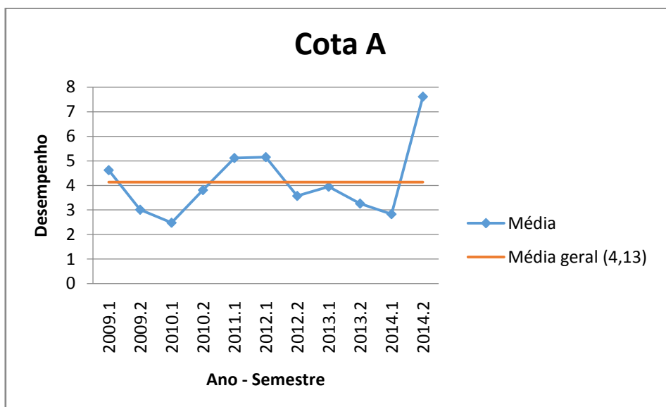
Figura 2 - Média do desempenho médio da Cota A- Química Industrial 2009 a 2014
