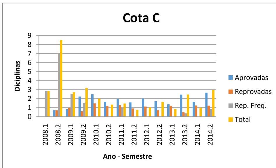
Figura 13 - Desvio padrão do número médio de disciplinas da Cota C- Química Industrial 2008 a 2014
