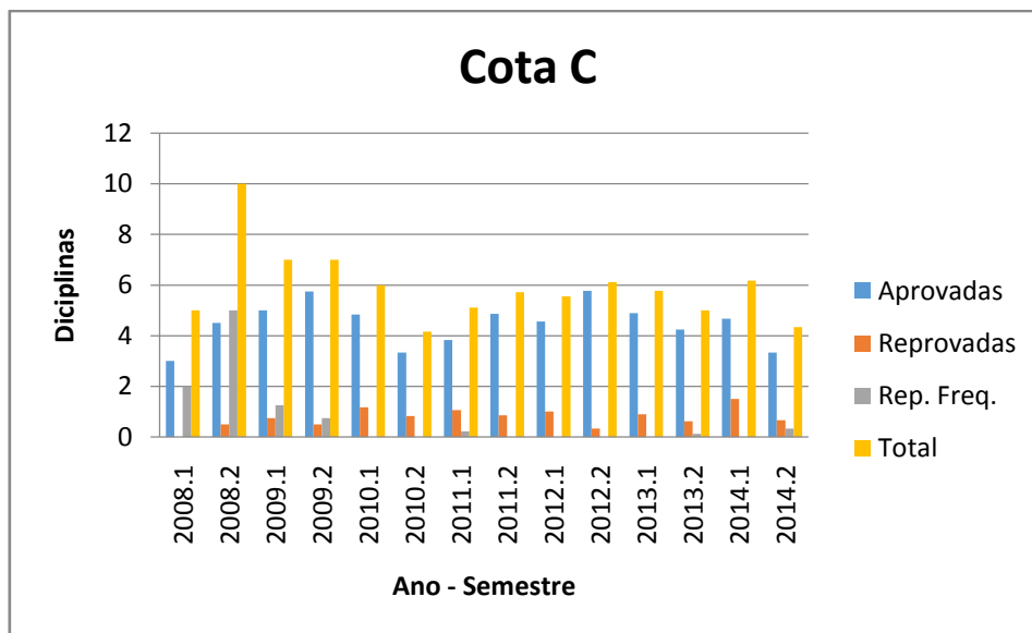
Figura 11 - Média do número médio de disciplinas da Cota C- Química Industrial 2008 a 2014
