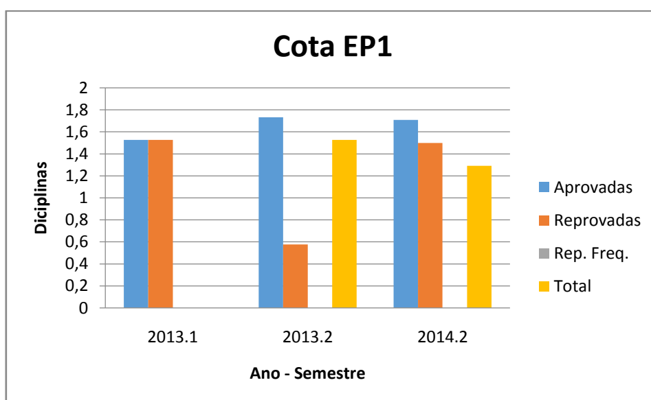
Figura 20- Desvio padrão do número médio de disciplinas da Cota EP1- Química Industrial 2013 a 2014
