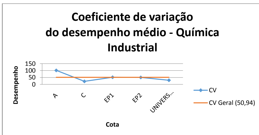
Figura 46 - Coeficiente de variação do desempenho médio do curso de Química Industrial no período de 2008 a 2014, pelas cotas
