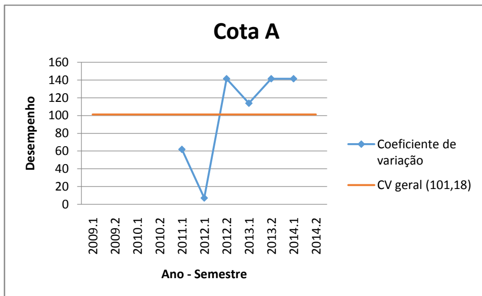
Figura 7 - Coeficiente de variação do desempenho médio da Cota A- Química Industrial 2009 a 2014
