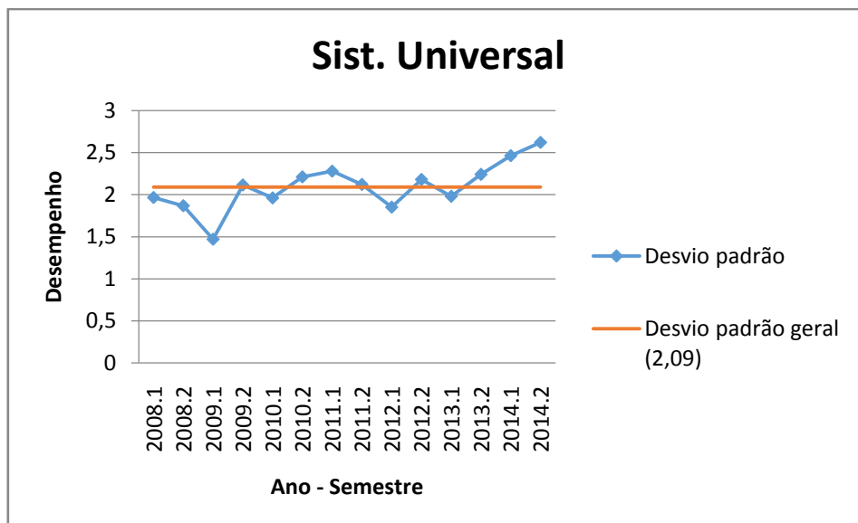
Figura 39 - Desvio padrão do desempenho médio do Sistema Universal- Química Industrial 2008 a 2014
