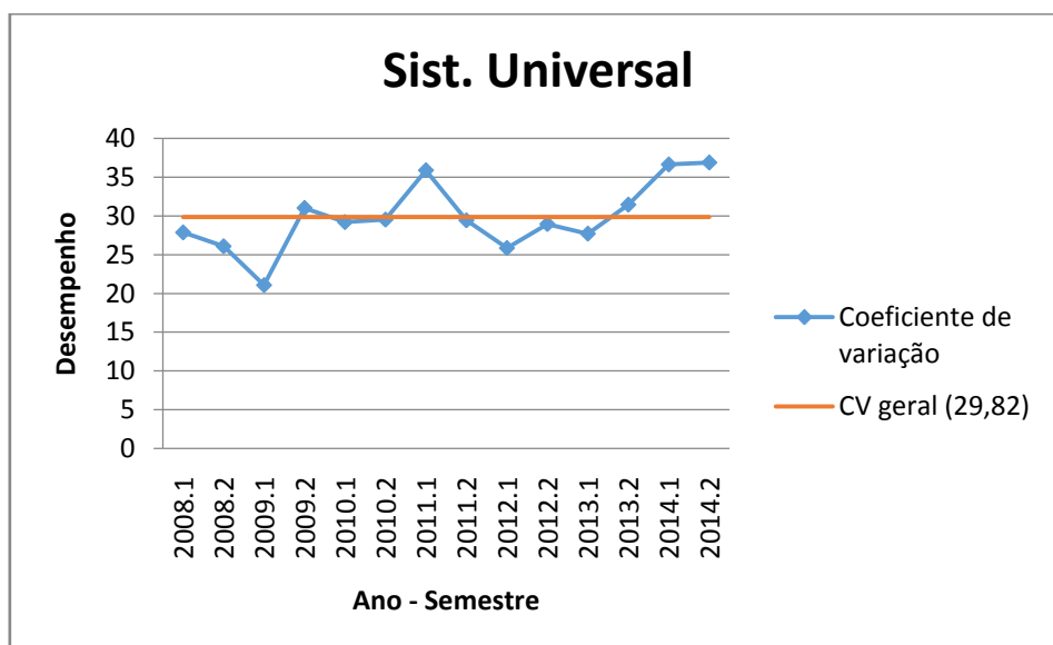
Figura 42 - Coeficiente de variação do desempenho médio do Sistema Universal- Química Industrial 2008 a 2014
