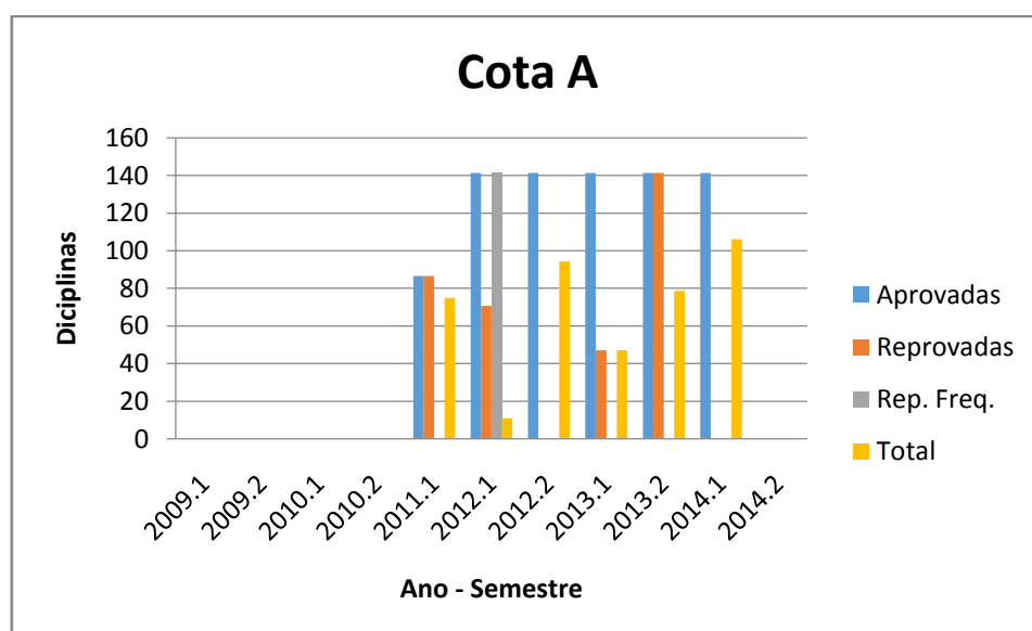
Figura 6 - Coeficiente de variação do número médio de disciplinas da Cota A- Química Industrial 2009 a 2014
