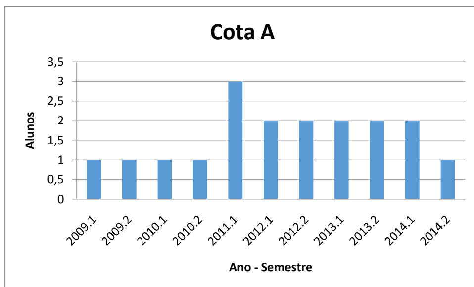
Figura 5 - Número de alunos da Cota A- Química Industrial 2009 a 2014
