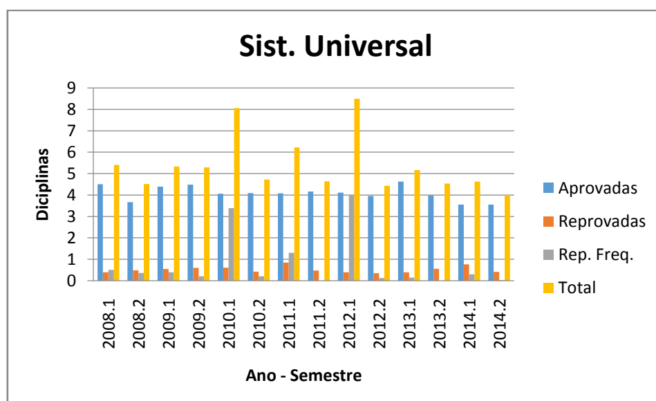
Figura 36- Média do número médio de disciplinas do Sistema Universal- Química Industrial 2008 a 2014
