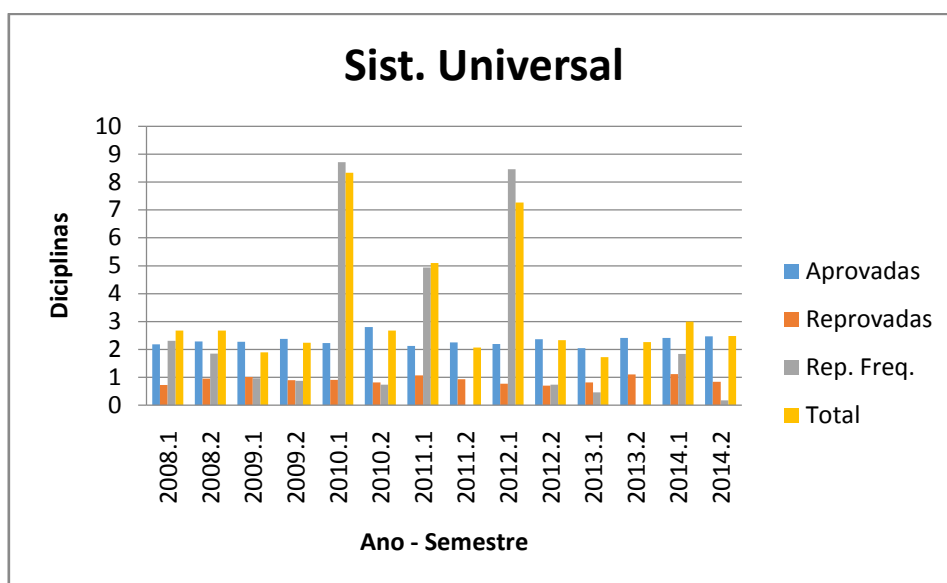
Figura 38 - Desvio padrão do número médio de disciplinas do Sistema Universal- Química Industrial 2008 a 2014
