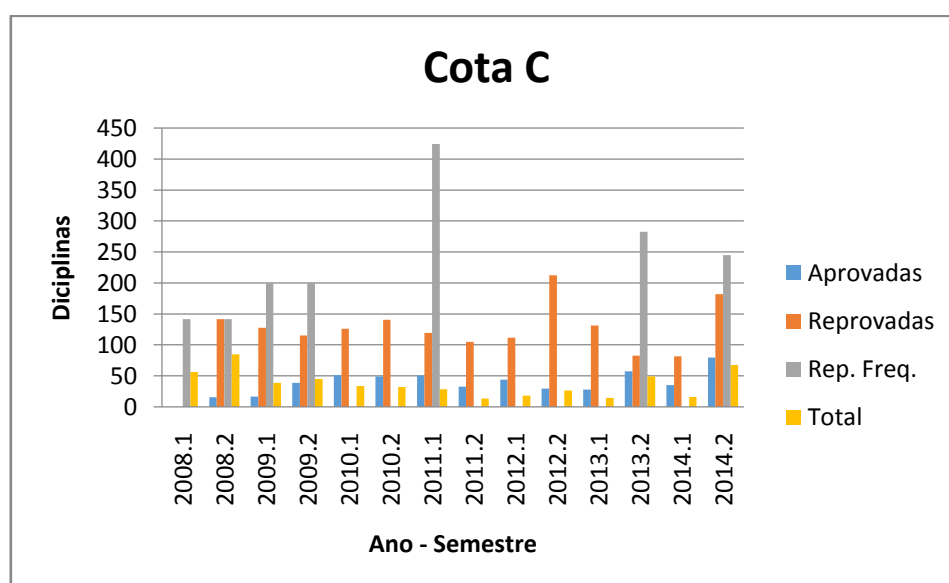
Figura 16 - Coeficiente de variação do número médio de disciplinas da Cota C- Química Industrial 2008 a 2014
