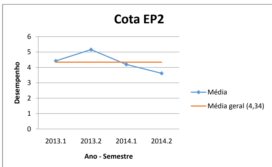
Figura 28 - Média do desempenho médio da Cota EP2- Química Industrial 2013 a 2014
