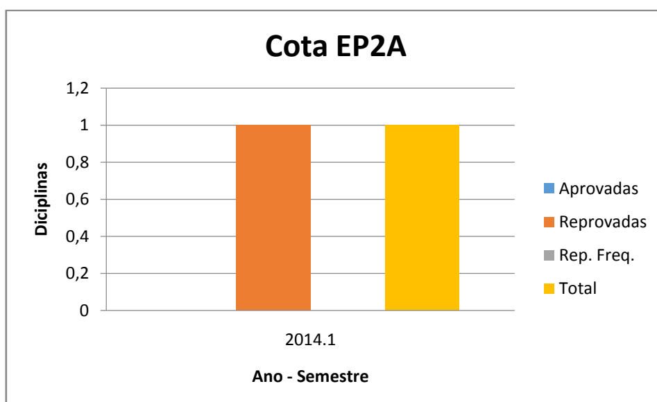
Figura 34- Média do número médio de disciplinas da Cota EP2A - Química Industrial 2013 a 2014
