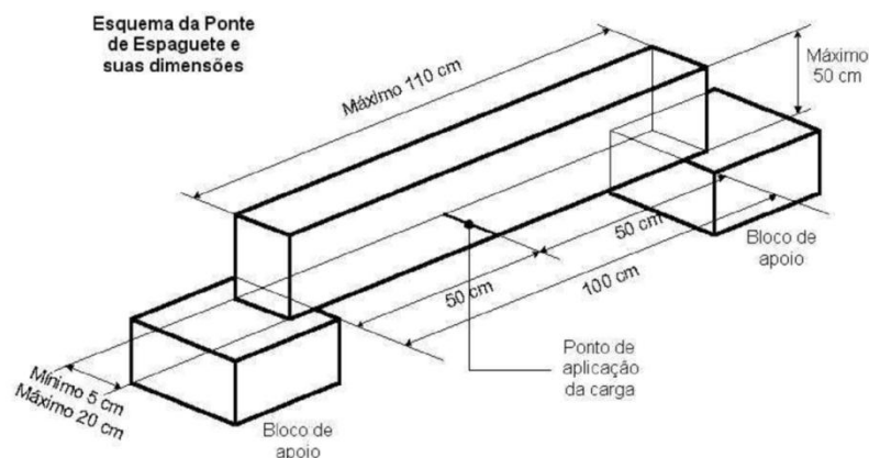
Figura 3. Disposição da ponte de espagete e suas dimensões.
